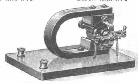
Nr. 1293. Dynamomaschine mit natürlichem Magnet, gute Leistungen; speist bis zu 2 Lampen à 4 Volt. Größe 10x15 cm. Stück Mk. 7.70
