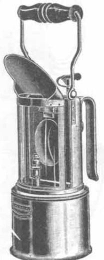
Nr. 2462. Azetylen-Grubenlampe,
