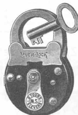
Nr. 4876. Vorhangschloß schweres, zweitouriges Schloß mit Zuhaltungen, federndem Verdeck und Ohrenverstärkung, schwarz emailliert, mit Messingbeschlag, Bügel blank geschliffen. Gewicht ca. 250 g. Mit 2 Schlüsseln. Stück 85 Pf.
