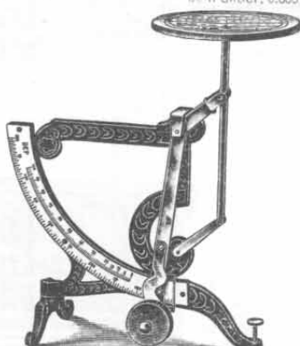
Nr. 533. Briefwaage in hübscher und starker Ausführung, bis 550 g wiegend. Mit weiß emaillierter Skala. Höhe 27 cm. Stück Mk. 3.75
