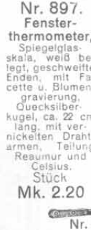
Nr. 897. Fensterthermometer, Spiegelglasskala, weiß belegt, geschweifte Enden, mit Facette u. Blumen gravierung, Quecksilberkugel, ca. 22 cm lang, mit vernickelten Drahtarmen, Teilung Reaumur und Celsius. Stück Mk. 2.20
