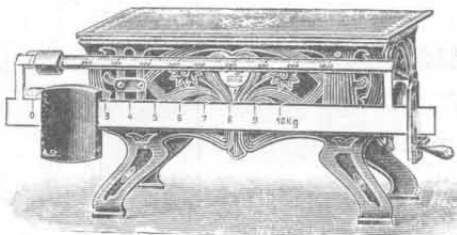
Nr. 5537. Laufgewichtswage, 10 kg Tragkraft, als zuverlässige Paket- und Haushaltswage besonders zu empfehlen, mit elegant dekorierter Eisenplatte, 20x30 cm groß. Die mittels Präzisions-Teilmaschine gravierten Laufgewichtslängen ermöglichen das Ablesen eines Gewichtes von 10 zu 10 g. Da die Pfannen und Messer aus bestem Stahl hergestellt sind, wiegt die Wage dauernd präzise. Stück Mk. 19.50
