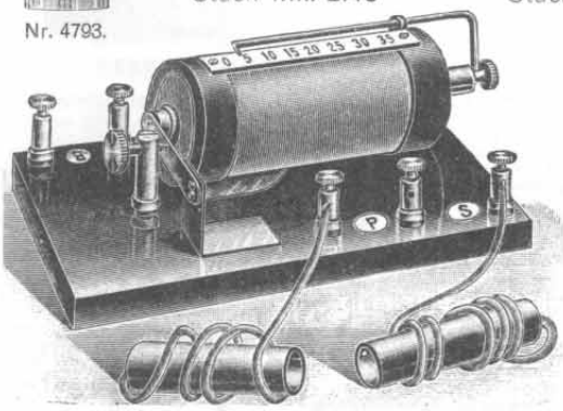
Nr. 2978. Induktionsapparat (Elektrisierapparat) auf schwarz emaillierter Metallplatte montiert. Alle übrigen Metallteile sind fein vernickelt. Mit Zelluloidskala und 3 Klemmen für P- und S-Strom, sauber und solide gearbeitet. Stück Mk. 2.80
