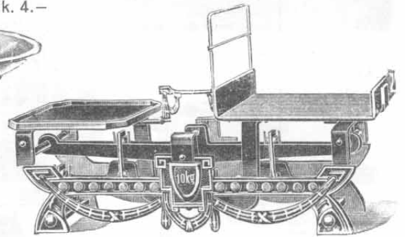
Nr. 6295. Tafelwage,
