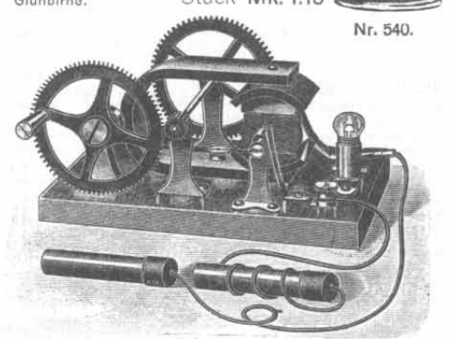
Nr. 9967. Elektrisiermaschine. Durch einfaches Drehen wird Induktionsstrom erzeugt. Auch läßt sich die Maschine zur Erzeugung von Licht verwenden. Mit zwei Handhaben und einer Glühlampe. Größe 13x8 cm. Stück Mk. 6.85
