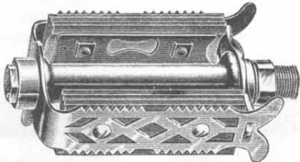
Nr. 1112. Sehr starkes Gummiflügelpedal für Tourenmaschinen, bequeme, nicht zu schmale Form. Konusse gehärtet, aus gutem Material, staubsicher und ölhaltend, sauber poliert und vernickelt. Zum Einschrauben, mit Rechts- und Linksgewinde. Paar Mk. 1.85
