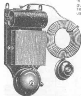
Nr. 2189. Klingelgarnitur. Vollständig montiert; bestehend aus: 1 Läutewerk mit 1 Trockenelement, 2 Anschlußklemmen, 10 m Doppelleitungsdraht, 1 Druckknopf und verzintene Haken. Komplett im Karton Mk. 3.—
