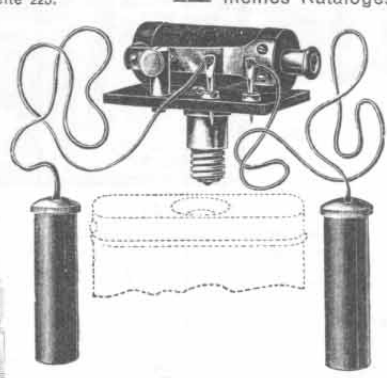
Nr. 1792. Elektrisierapparat. Dieser Elektrisierapparat ist der kleinste Apparat der Welt und wirkt genau so kräftig wie jeder größere teure Apparat. Der Elektrisierapparat kann nach Entfernung der Glühbirne an deren Stelle auf jede beliebige Taschenlampe der Seite 226 meines Kataloges aufgeschraubt werden, wodurch dann der Apparat gebrauchsfertig ist. Ohne Taschenlampe. Stück Mk. 2.40
