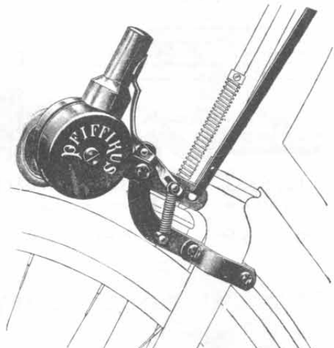
Nr. 1248. Radlaufpfeife „Piffikus“.
