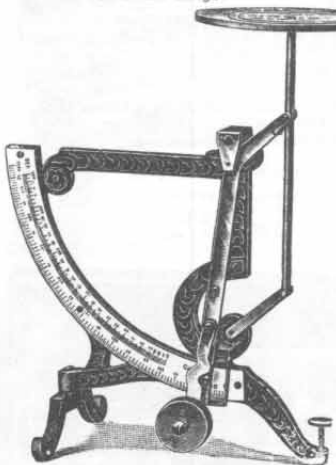
Nr. 531. Briefwaage, extra groß, bis 1000 g wiegend, in fein schwarz lackierter und vernickelter Ausführung, mit weiß emaillierter Skala. Höhe 35 cm. Stück Mk. 7.50
