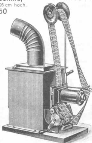
Nr. 9970. Kinematograph. Für 3,5 cm Glasbilder, gute Ausführung. Beigegeben: 3 farbige Filme, 6 lange Glasbilder, 5" Flachbrennvorlampe. Stück Mk. 6.75
