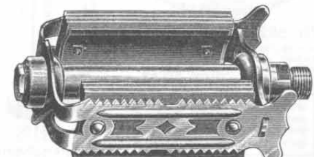
Nr. 3472. Extra breites, doppelstaubsicheres Gummiflügelpedal, welches infolge der stabilen Ausführung als Tourenpedal besonders zu empfehlen ist. Dasselbe hat auf der Achse eine besondere Staubkapsel, wodurch größtmögliche Staubsicherheit erreicht wird. Die Konusse und Achsen sind bestgehärtet, sauber und exakt gearbeitet, in fein vernickelter Ausführung. Zum Einschrauben, mit Rechts- und Linksgewinde. Paar Mk. 2.30
