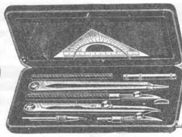
Nr. 9586. Reißzeug, geeignet für Schüler höherer Lehranstalten u. Fortbildungsschulen. Ganz vorzüglich gearbeitet. Das Reißzeug ist in einer großen Anzahl von Schulen behördlich eingeführt. Aus gezogenem Messing mit Stahlspitzen. In feinem Etui, innen blau Samt, außen schwarz Viktorialeder. Stück Mk. 4.50
