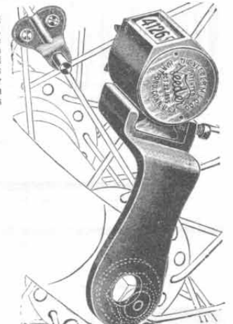
Nr. 1363. Kilometerzähler für Motorräder.
