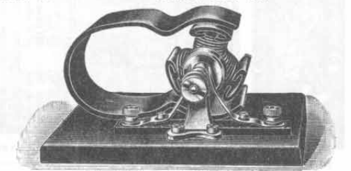
Nr. 5813. Elektromotor. Billig und doch solid. Außerst kräftig, mit dreifachem T-Anker und natürlichen Magneten, wodurch der Motor in jeder Stellung von selbst anläuft. Sehr gut zum Auseinandernehmen geeignet. Stück Mk. 1.90
