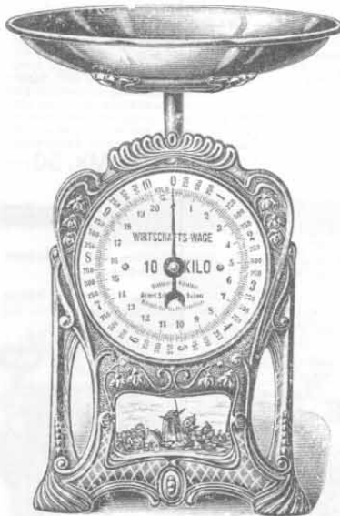
Nr. 5228. Wirtschaftswage, 10 kg genau wiegend, ganz neue Ausführung und besonders schön dekoriert; unten mit echter Steinguteinlage. Das Zifferblatt ist echt emailiert, der Zeiger kann mittels Regulierschraube stets auf 0 ausgerichtet werden. Stück Mk. 3.40
