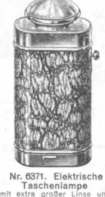
Nr. 6371. Elektrische Taschenlampe mit extra großer Linse und Metallfadenlampe ausgestattet. Die Hülse ist fein vernickelt und im mittleren Teile mit krokodilartigem Kaliko bezogen. Mit Dauerkontakt. Größe 105x45x24 mm. 2,5 Volt. Stück Mk. 1.85
