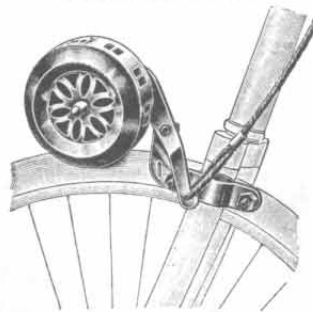
Nr. 5588. Radlauf-Torpedopfeife mit Antrieb durch das Vorderrad. Aus Stahl, vernickelt, mit emailliertem Halter zum Anbringen an der Vordergabel und mit Gummi überzogener Welle. Letztere ist auf Kugeln gelagert, daher leichter Lauf. Durchdringender pfeifender Ton, ähnlich einer Schiffssirene. Durchmesser des Körpers 80 mm. Gewicht ca. 280 g, mit ca. 60 cm langer Schnur.
