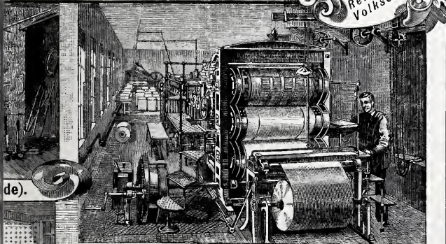
Rotationsmaschine.
