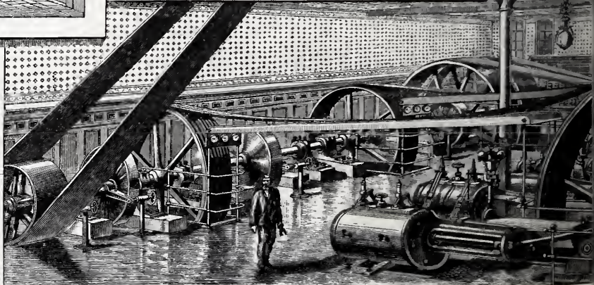
Dampfmaschinen- und Lichtmaschinenraum.
