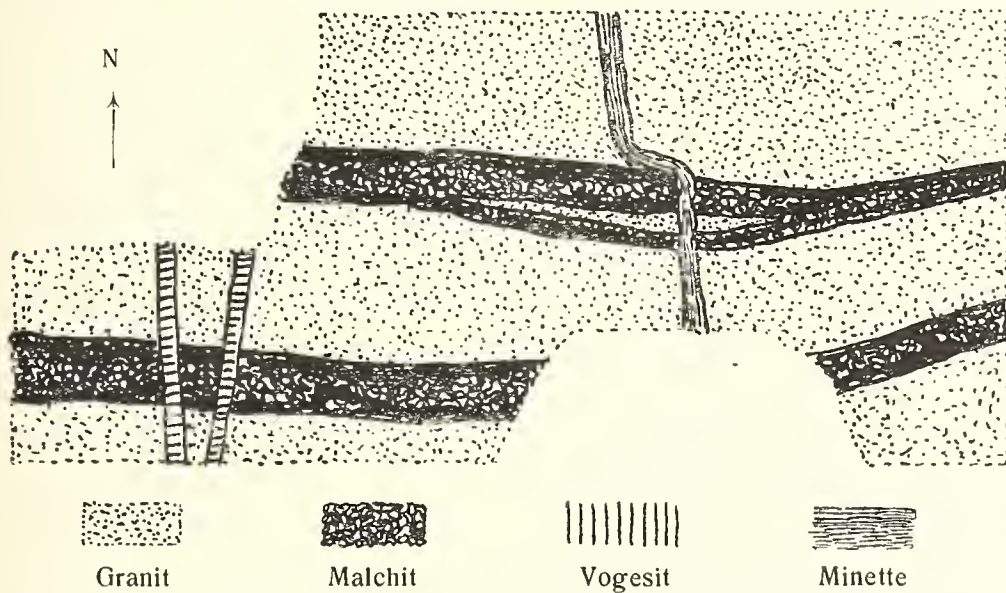
Abb. 5. Grundriß des Aufschlusses im Weidental am Südabhang des Luzibergeres.
