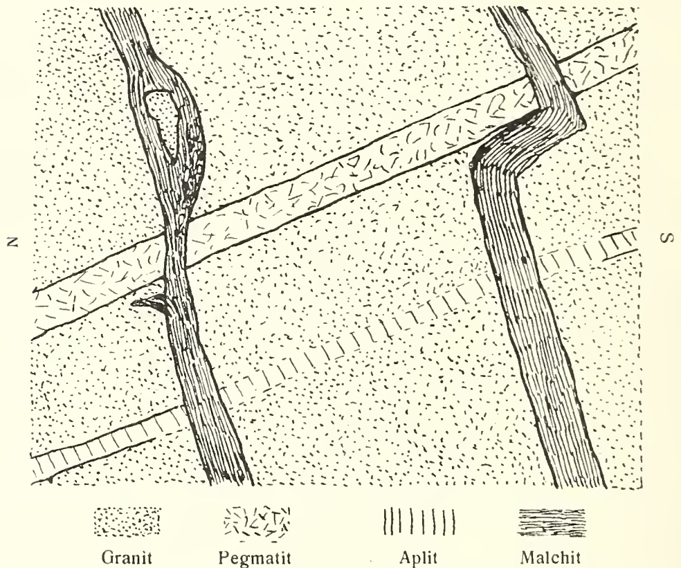
Abb. 2. Durchbruch zweier Malchitgänge durch einen Aplit- und einen Pegmatitgang im Alsbacher Gemeindebruch.
