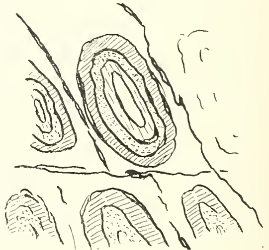
Abb. 7. Auf einer Kluff des Malchits von Messel (nördlich von Darmstadt) vorgezeichnete Brotlaibformen.
