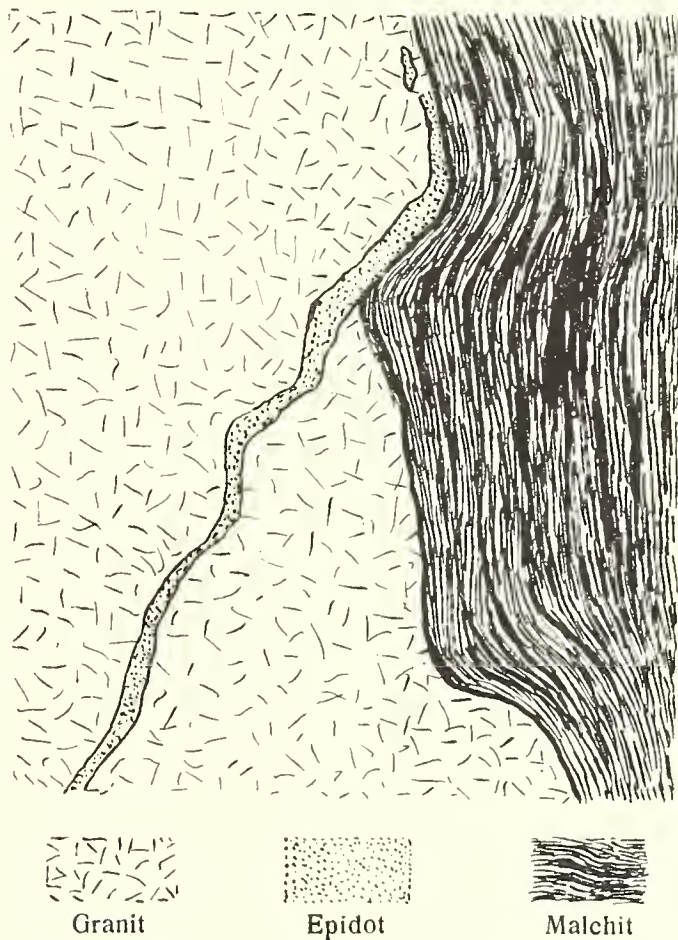
Abb. 11. Scharung eines Epidotganges mit Malchit. Bruch der deutschen Steinindustrie, A.-G., am Luzenberg. (Handstück.)
