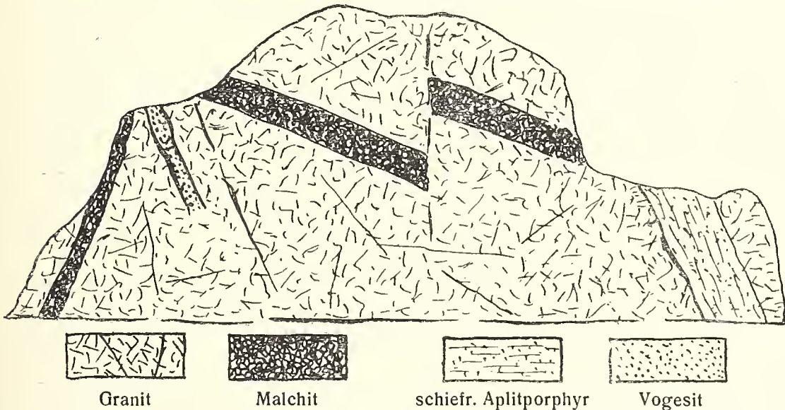
Abb. 9. Verwerfung eines Malchitganges im Südbuch der Steinwerke „Melibokus“ am Luziberg. (Die Sprunghöhe beträgt etwa 3 m).
