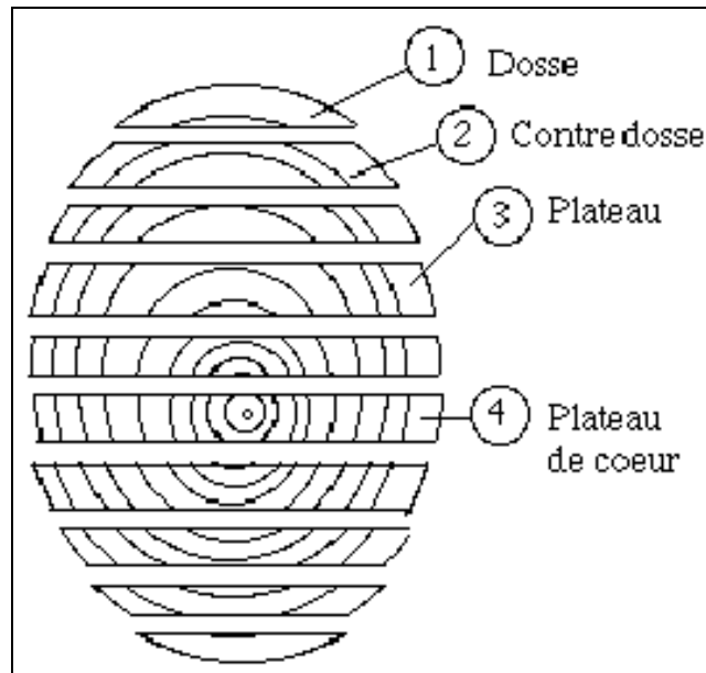
Figure n°1: Débit d'une grume en plot.
