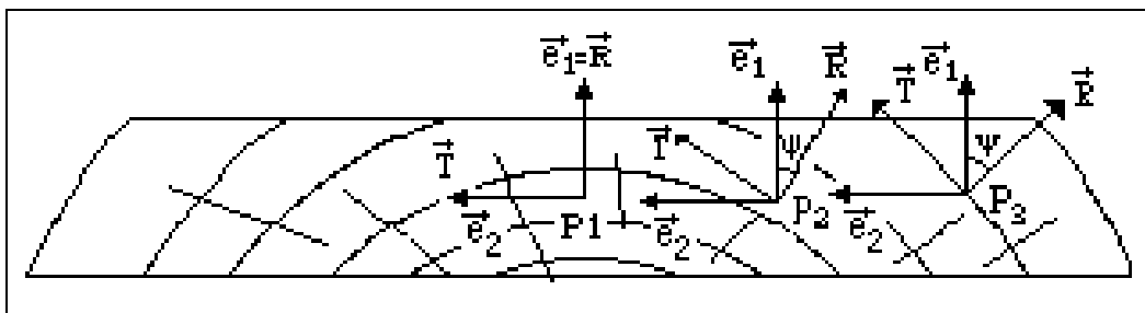
Figure n°2: Evolution spatiale de l'orientation relative du repère de structure par rapport au repère matériel dans une contredosse.
