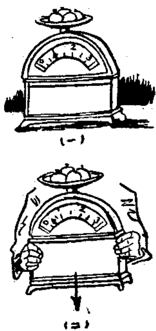
圖五 (一)四隻蘋果秤秤剛一磅 (二)但我把磅秤拿得很快的向下，磅秤上的指針，便退到零上來了
