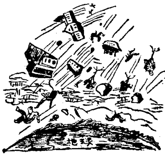
圖九 沒有地心吸力的世界，一切東西都被地球旋轉時所發生的離心吸力擲到空中去了。
