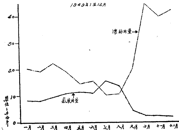
圖12 本市製水氣液漂粉用量消長比較
