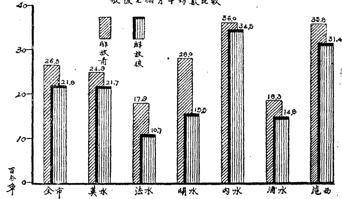
圖14 本市解放前後漏失水量比較
