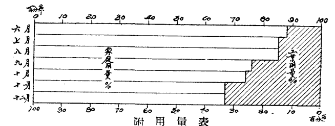
圖17 解放後本市煤氣用途分析 1949年6至12月
