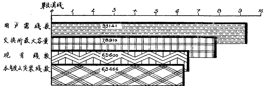
圖 19 上海電話公司機線容量使用情形
