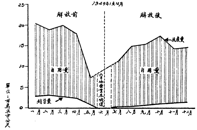
圖18 吳淞煤氣廠煤氣產銷情況 1949年1至12月
