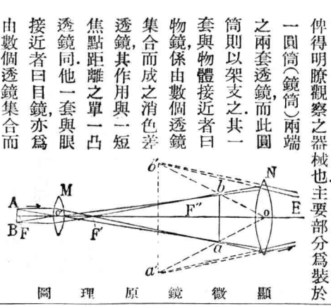
顯微鏡原理圖
