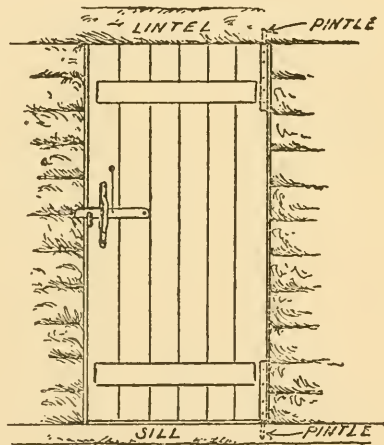
Fig. 276. The Door Hinges.
