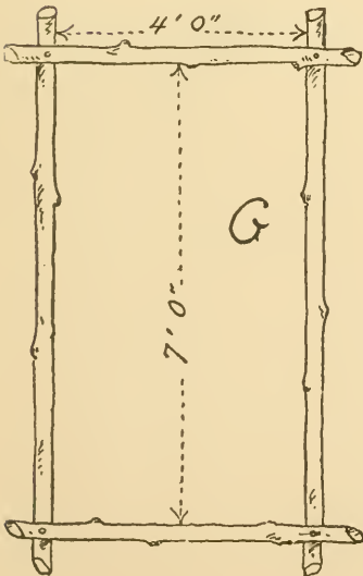
Fig. 311. G Frame (make two).
