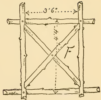
Fig. 310. F Frame (make two).
