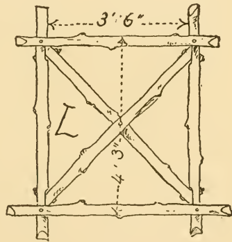
Fig. 316. L Frame (make two).
