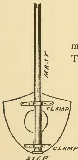
Fig. 117. The Mast Step.
