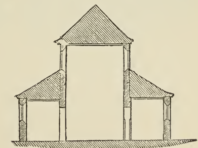
373. Plan and Section of Basse Œuvre, Beauvais. (From Woillez, "Monuments Religieux de Beauvais.")
