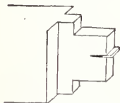
Fig. 97.—Foxed Tenon.
