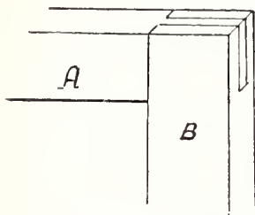
Fig. 92.—Mortise and Tenon.
