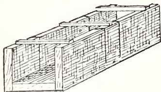
Fig. 56.—Mitre Box.
