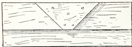
Fig. 53.—Mitre Shoot.
