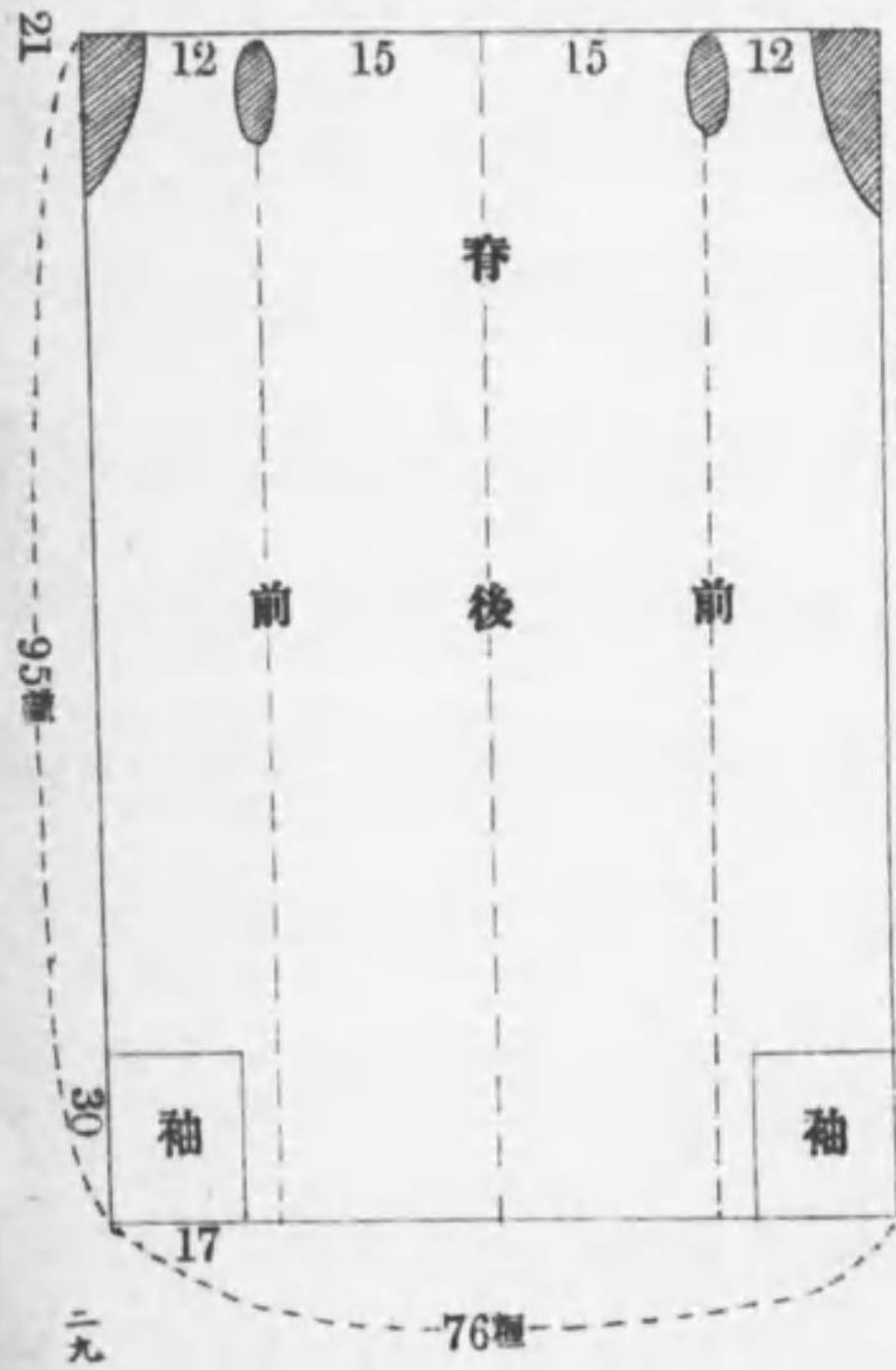
圖三第 方裁着下
