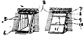
開啓時情形 關閉時情形 突出的入口
