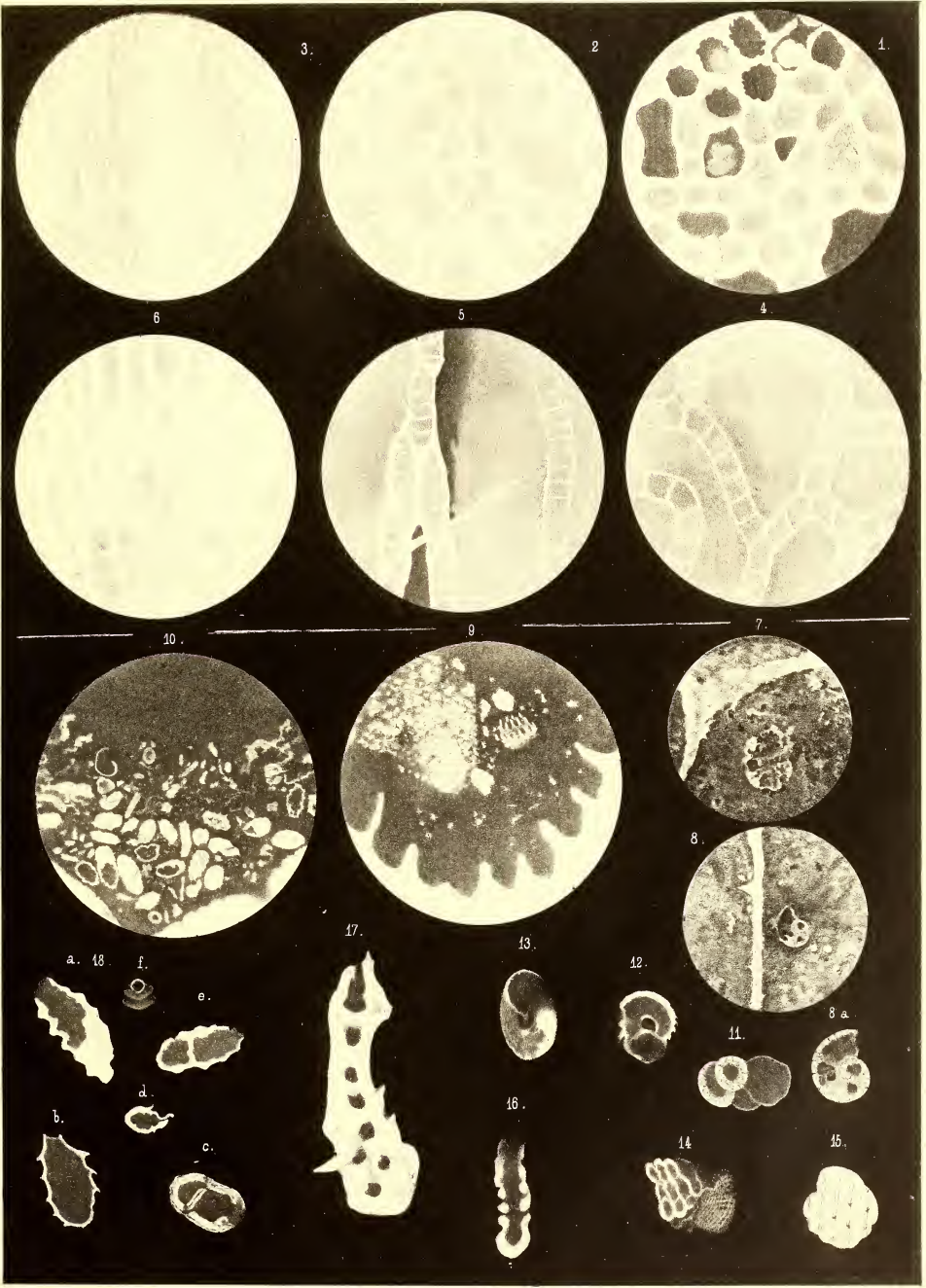
Silur. Foraminiferen
