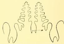
Fig. 22. M. Orbignyana .
