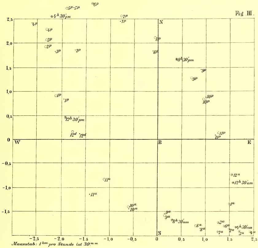
DIE LAGE DER ZERSTREUUNGS-AXEN UND DIE GRÖSSEN \frac{1}{k^2} UND \frac{1}{k_2^2} FÜR VERSCHIEDENE STUNDEN IN JULI 1886.
