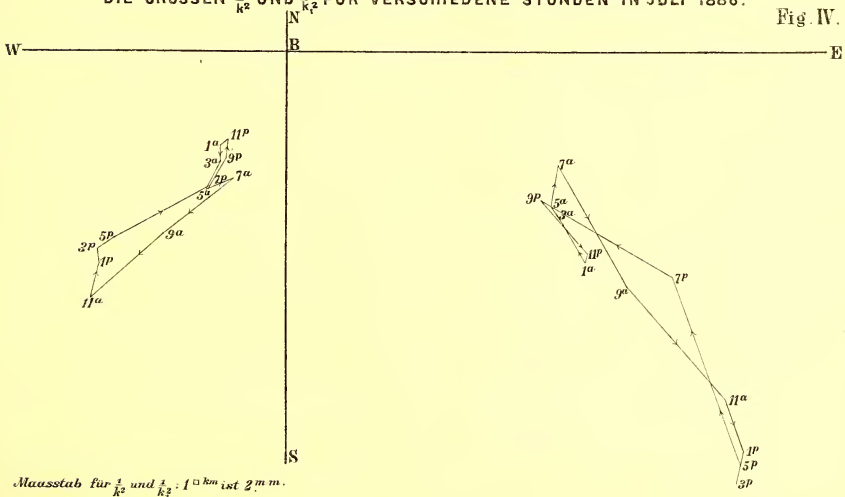
DIE LAGE DER ZERSTREUUNGS-AXEN UND DIE GRÖSSEN \frac{1}{k^2} UND \frac{1}{k_2^2} FÜR VERSCHIEDENE STUNDEN IN JULI 1886.
