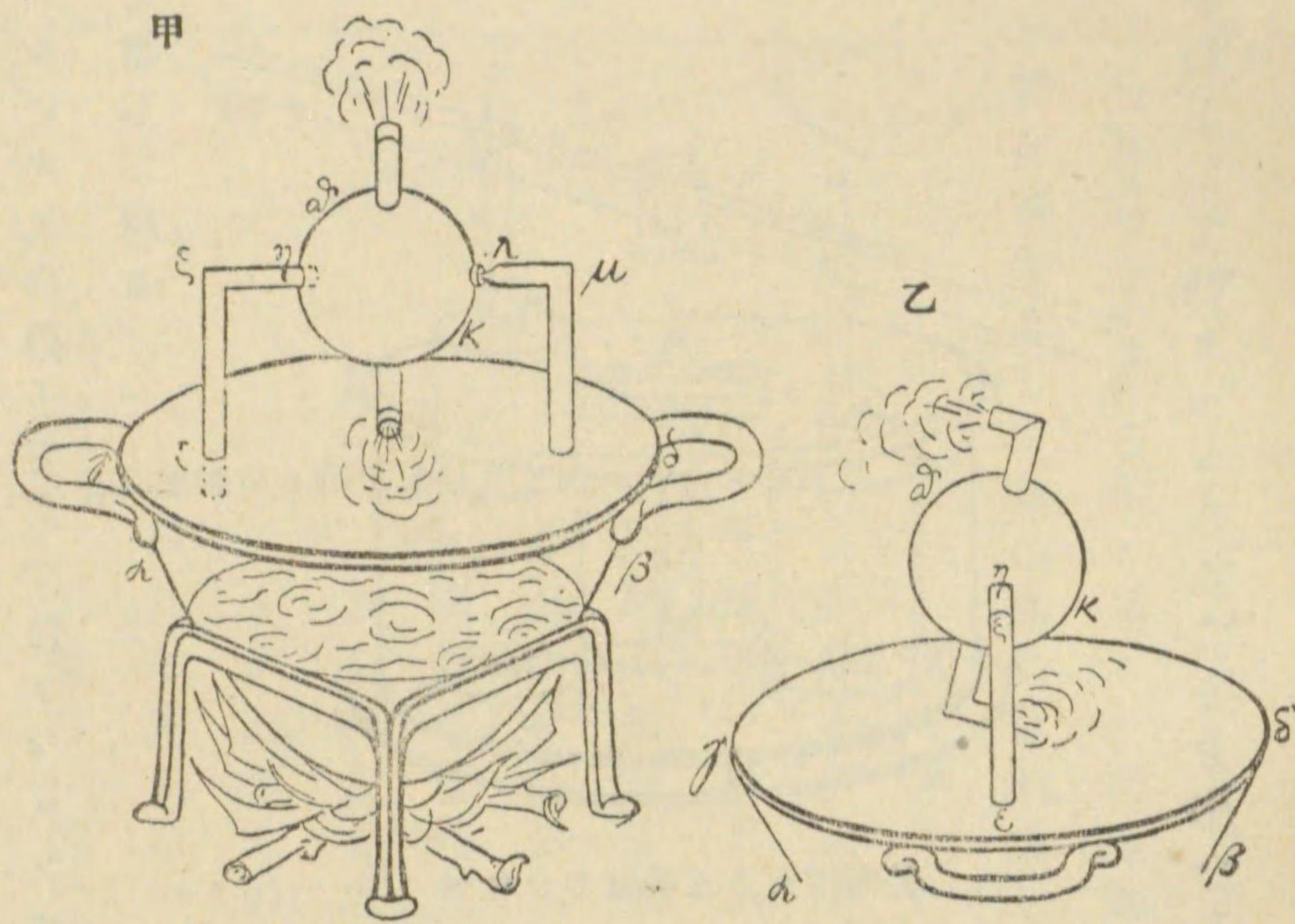
ヘロンの蒸気機関、甲正面圖、乙側面圖
