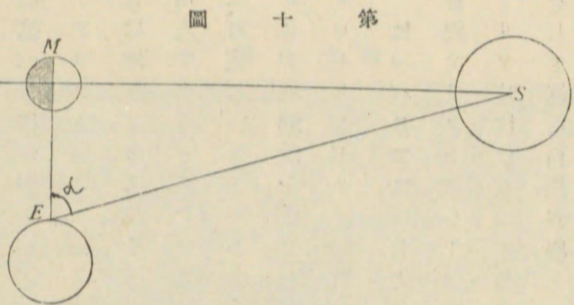
アリストタルコスの太陽と月の距離測定法 太陽……S 地球……E 月……M
