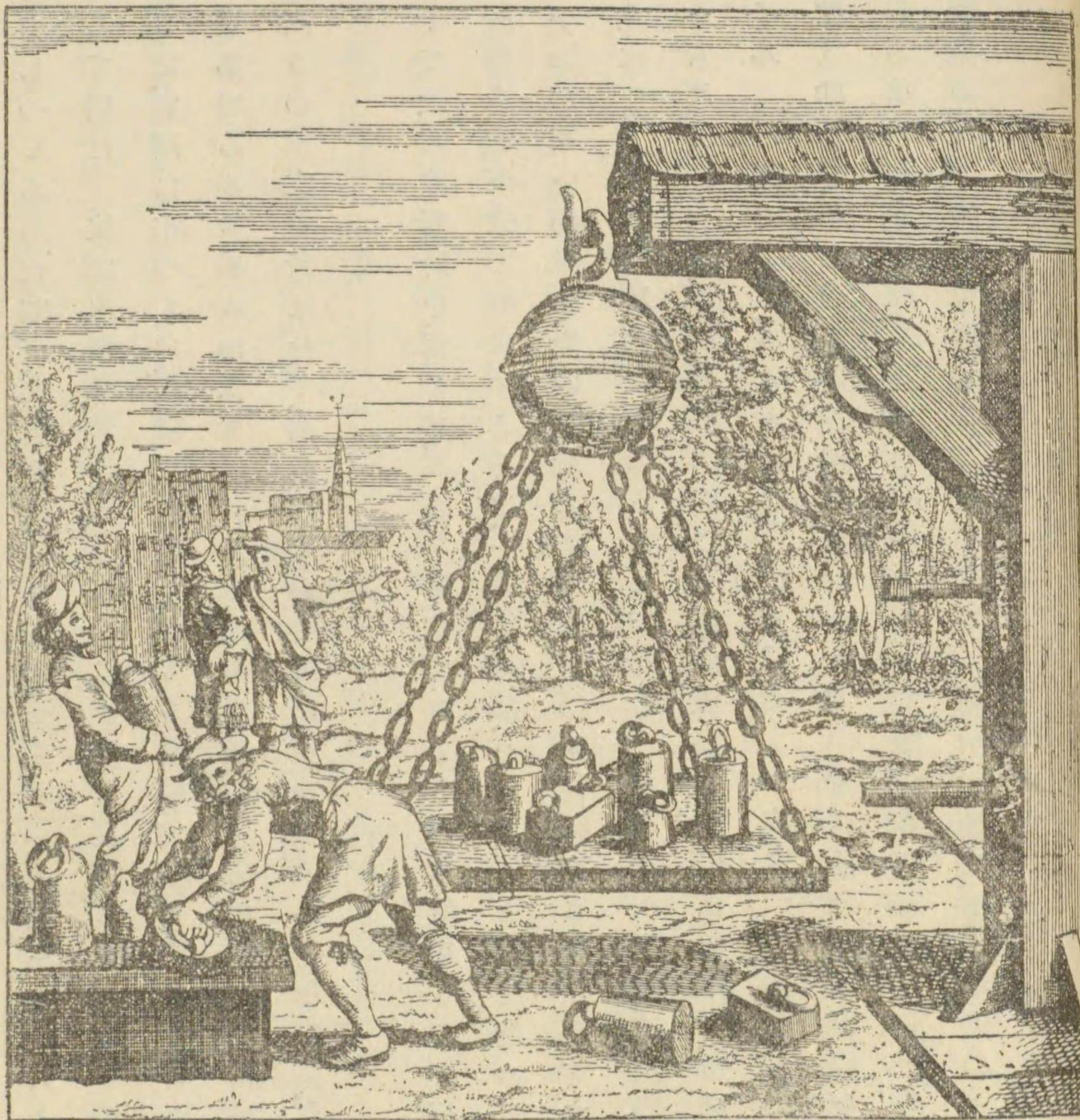
空眞で筒唧氣空のケリエゲ)球半のゲルブデグマ (す示をとこいなれ離に易容が球各の球たれさに
