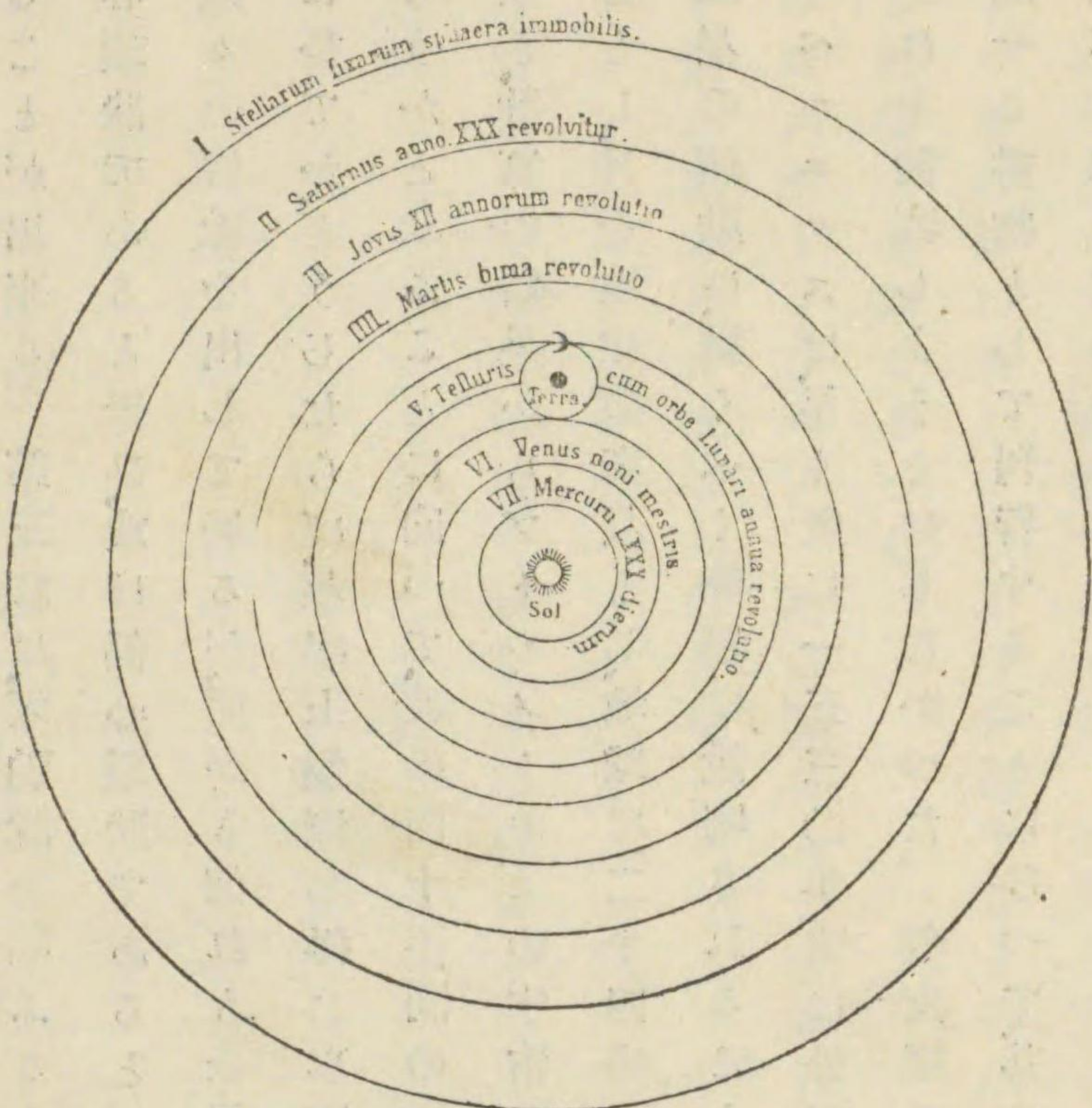
系宙宇のスクニルペコ (載轉らか「動運の體天」著のスクニルペコ)
