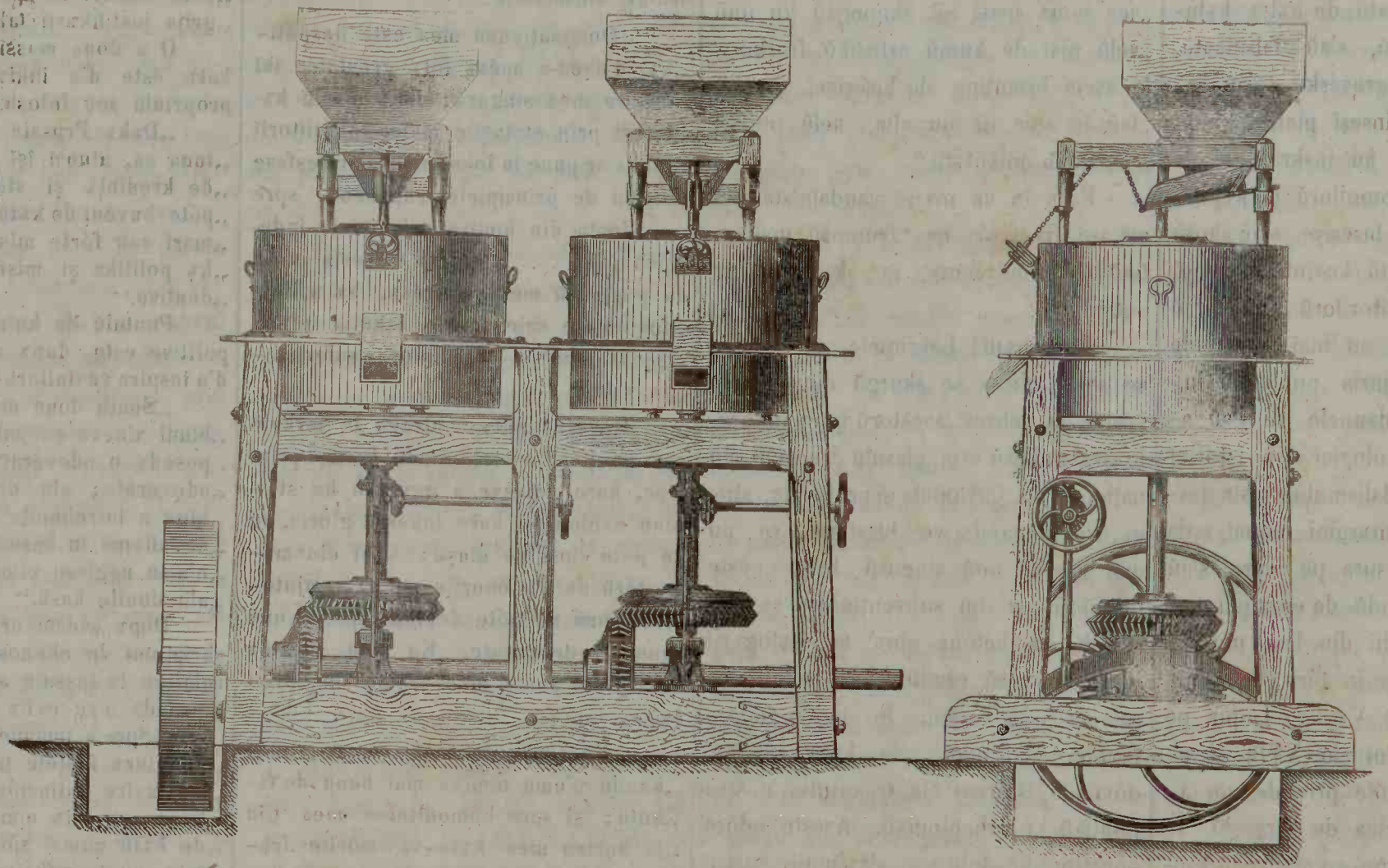
Moara de măcinat dublă perfecționată.
