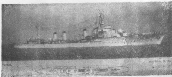
法國驅逐艦「威實」號
