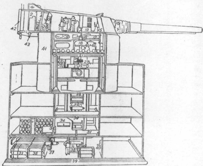
大砲構造之剖解
