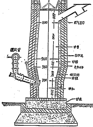
芙蓉鐵廠白煤煉鐵矮高爐示意圖 (1) 爐口中心直徑為4.0公尺，爐口中心直徑為5.7公尺，預備爐口直徑為4.0公尺，爐口中心直徑為4.0公尺。 (2) 爐內全部用耐火磚，爐內鋪設耐火磚，爐內鋪設耐火磚，爐內鋪設耐火磚。
