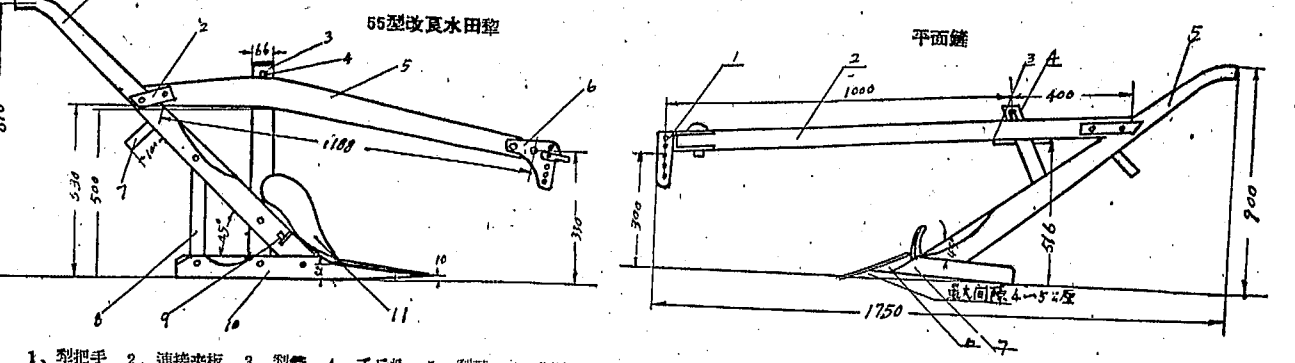
1. 犁把手 2. 连接板 3. 犁轡 4. 千斤 5. 犁铧 6. 深沟调节板 7. 扶手 8. 犁铧注 9. 犁铧注 10. 犁铧注 11. 犁头
