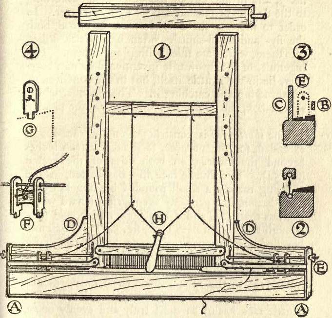
FIG. 54.—Fly-shuttle Batten.
