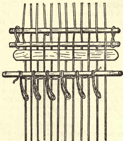
FIG. 40.—Headle Rod.
