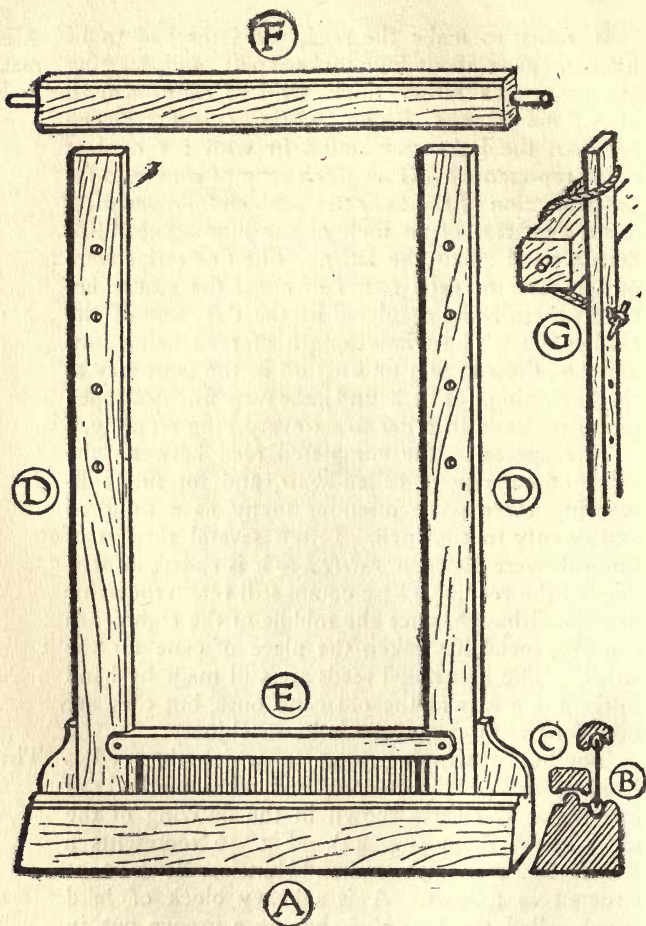
FIG. 46.—Hand-batten.
