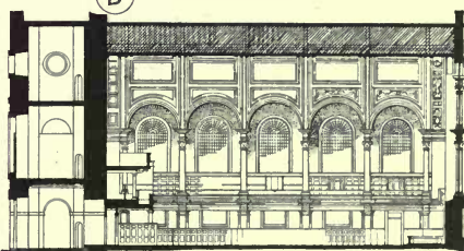
D LONGITUDINAL SECTION
