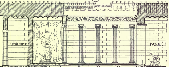
(D) LONGITUDINAL SECTION SHOWING THE CELLA & ANTIUM, OPISTHODOMUS & PRONAOS.
