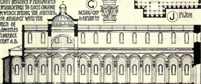
(K) LONGITUDINAL SECTION
