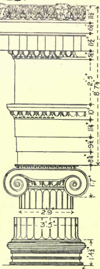
(D) ENLARGED CAPITAL, BASE AND ENTABLATURE
