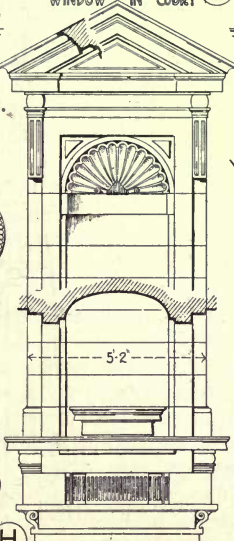
H NICHE, MERCATO NUOVO.
