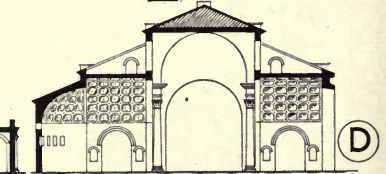
BASILICA MAXENTIUS, TRANSVERSE SECTION.
