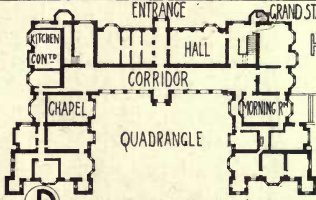
(D) GROUND FLOOR PLAN
