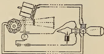
Telephote.
