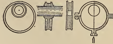
Eccentric.
