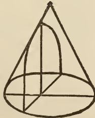
Hyperbola.
