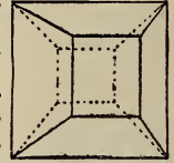
Decahedron.
