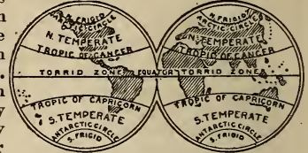
The Zones.
