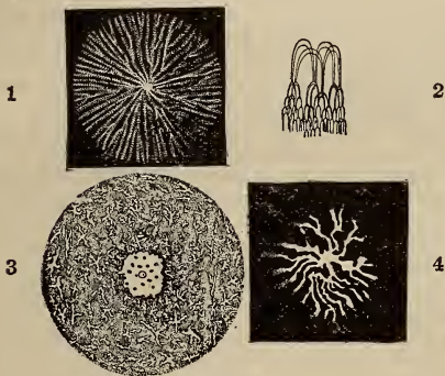
Cohesion Figures.
