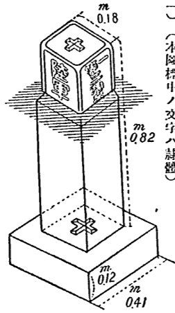
一等三角點石標
