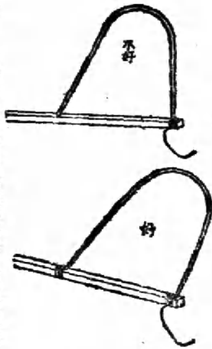
第三十圖 尾翼捆綁法
