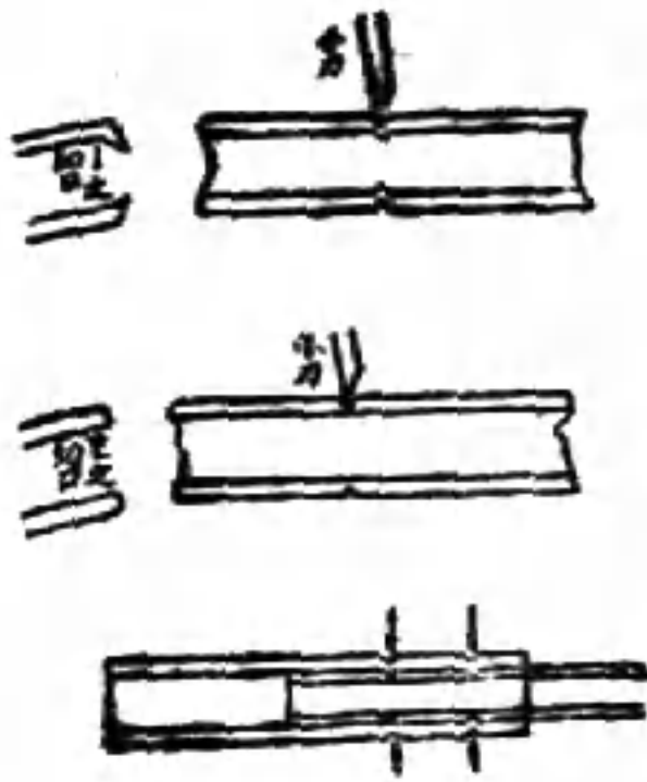
第八圖 鉛管嘴切斷及連接法
