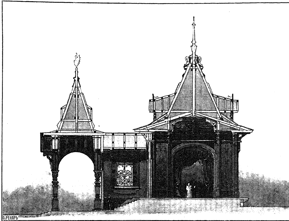
Платформа для Императорскаго поѣзда на вокзалѣ Московско-Брестской ж. д. (разрѣзъ).
