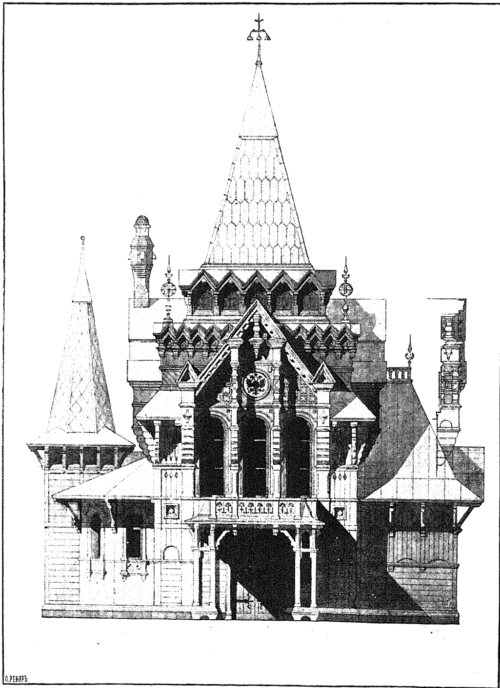
Павильонъ на ст. „Одинцово“.
