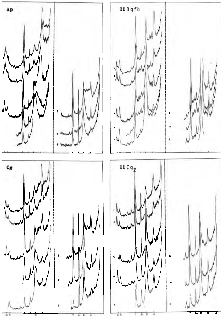
Figure 1 a. Diffractogrammes obtenus pour certains horizons de la série Chaloupe après aitements suivants : 1) saturation au Ca ; 2) Ca + glycérol ; 3) saturation au K ; 4) K + ; 5) K + 550°C ; 6) citrate de Na + K ; 7) cit. + K + 400°C ; 8) cit. + K + 550°C.
