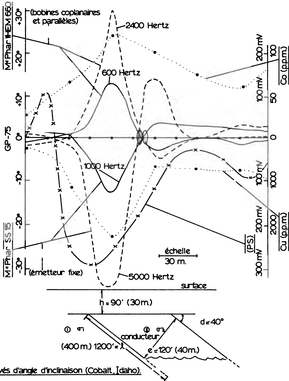
Figure 3. Profils typiques de la variation de l'angle d'inclinaison (EM), de la différence de potentiel (PS) et de la concentration en cuivre et cobalt dans les sols (ppm) au-dessus d'une lentille minéralisée (remplacement); il s'agit ici d'une extension de la zone minéralisée: Dandy.
