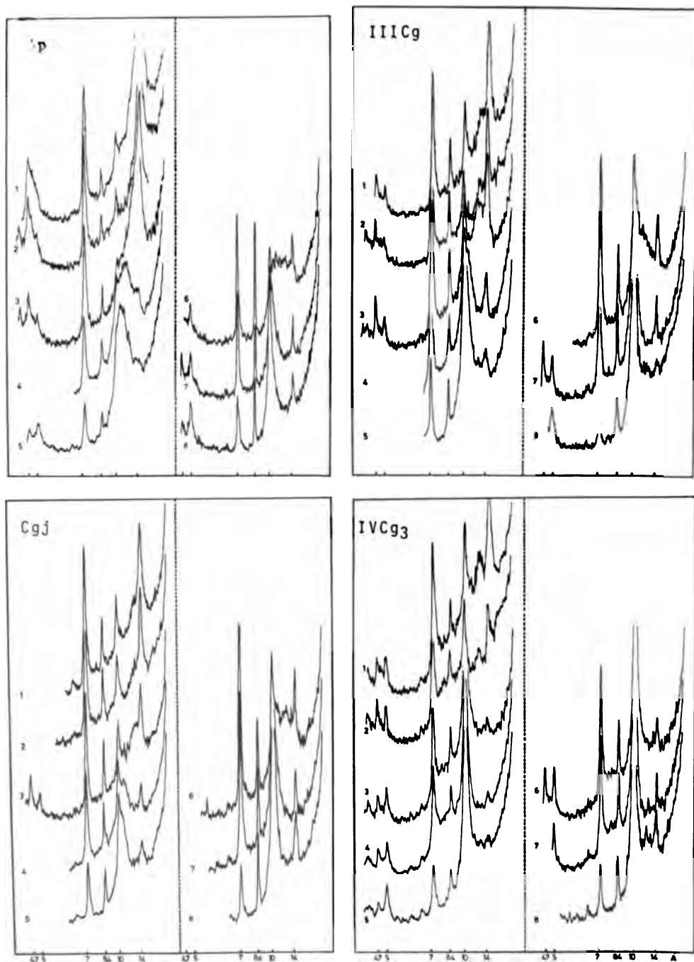
Figure 1 b. Diffractogrammes obtenus pour certains horizons de la série Batiscan après les traitements suivants : 1) saturation au Ca ; 2) Ca + glycérol ; 3) saturation au K ; 4) K + 400°C ; 5) K + 550°C ; 6) citrate de Na + K ; 7) cit. + K + 400°C ; 8) cit. + K + 550°C.
