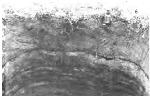
Figure 6. La série Hanni avec couverture récente de sable éolien. Noter les ferruginisations stratiformes et en plaques.
