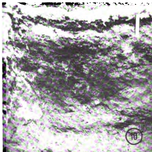
Figure 10. La série Josua : podzol humo-ferrique avec induration dans l'horizon Bf.
