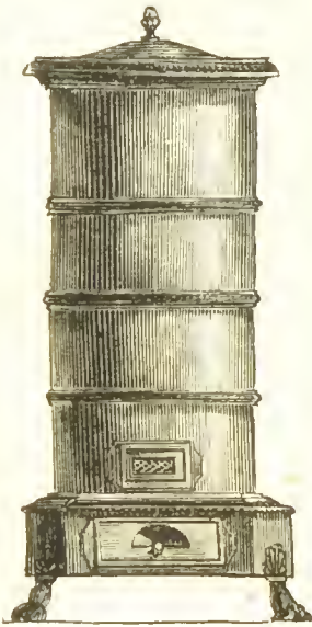
Grav. 78. — Poêle à coke.
