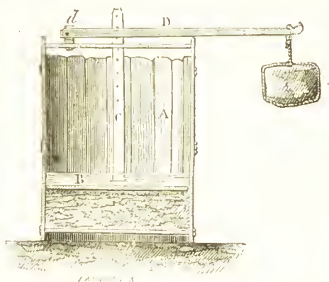
Grav. 105. — Coupe de la presse à choucroute.
