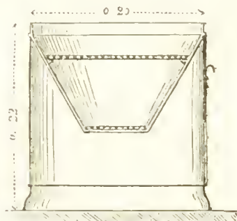
Grav. 36. — Coupe du fourneau portatif.
