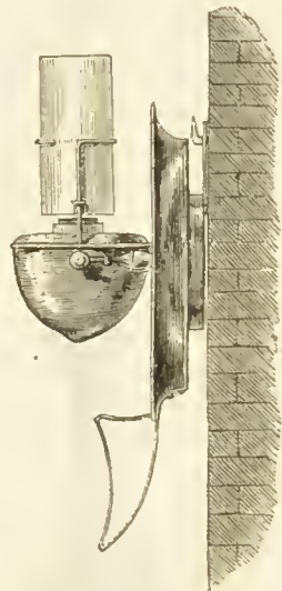
Grav. 84. — Lampe à bascule suspendue.
