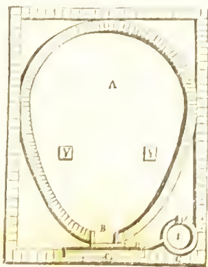
Grav. 98. — Four.
