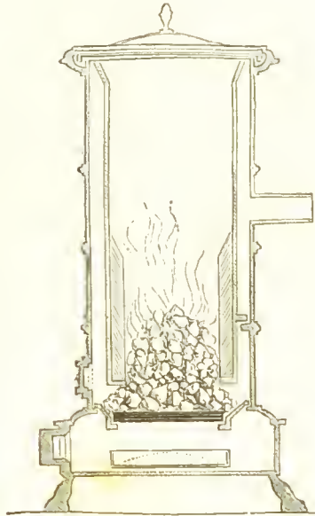
Grav. 79. — Coupe du poêle à coke.
