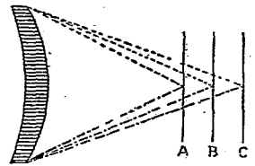
有色光差鏡頭 第四圖
