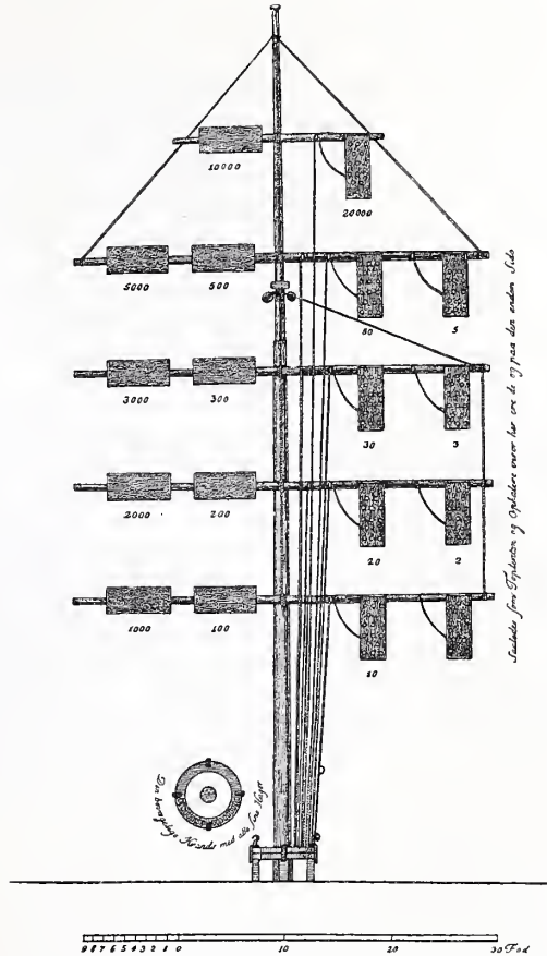
Optisk Telegraf (dansk System).
