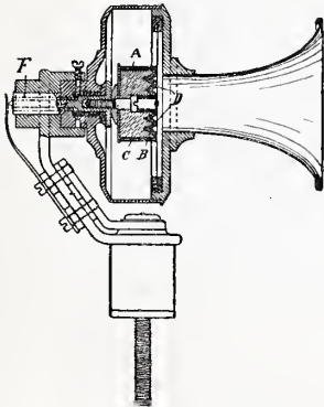
Ericssons Kulkornsmikrofon.
