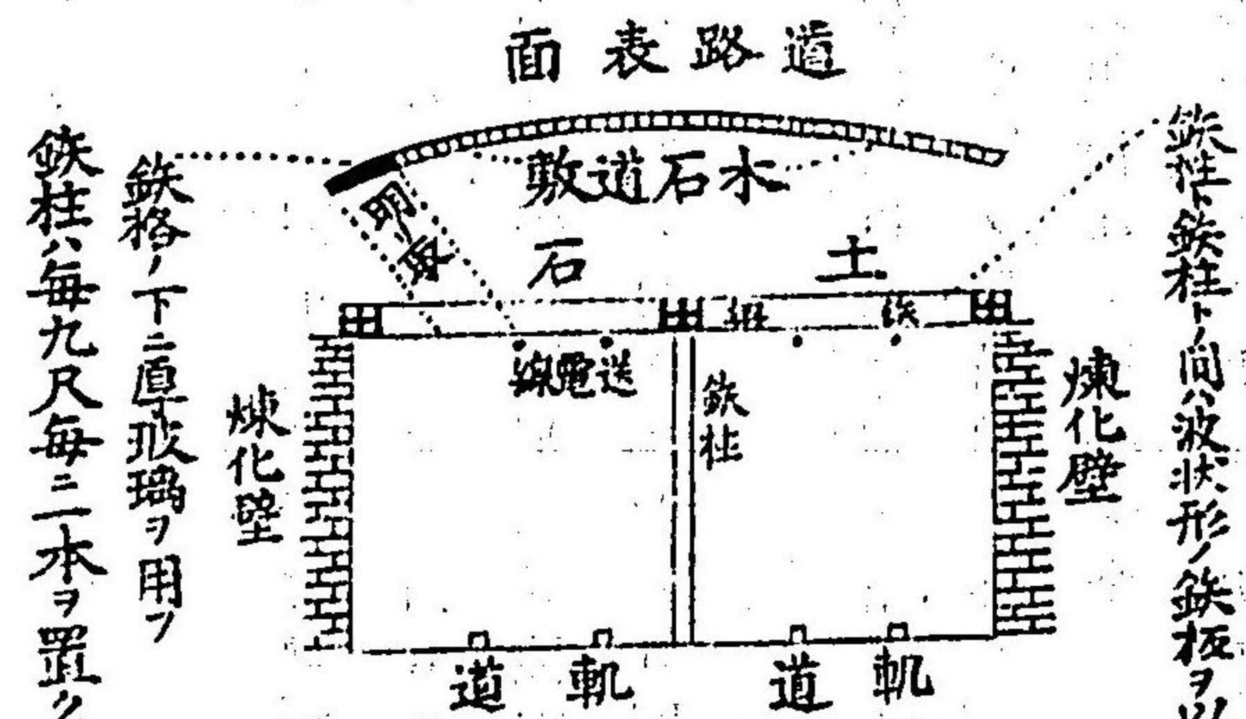
以上ハ停車場外ノ鐵道斷面略圖ナリ
