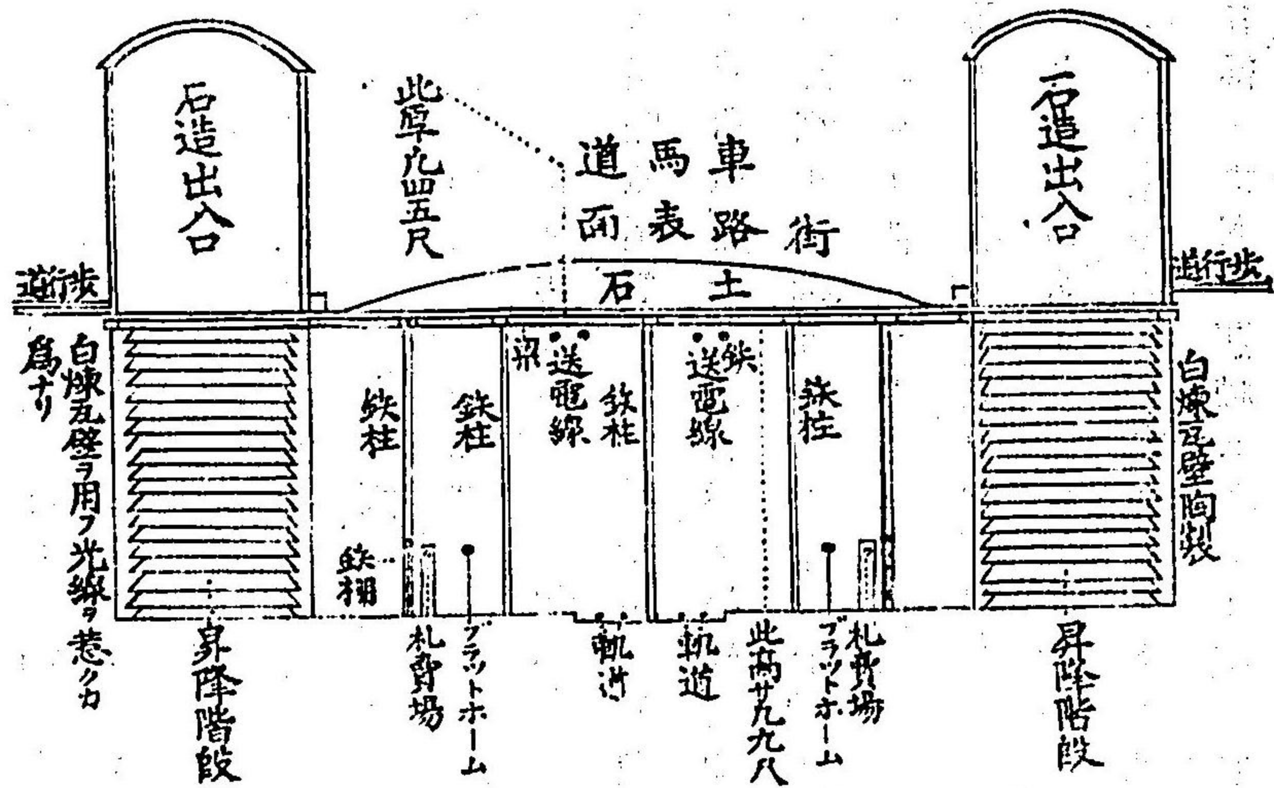
以上ハ停車場内ノ略圖ナリ
