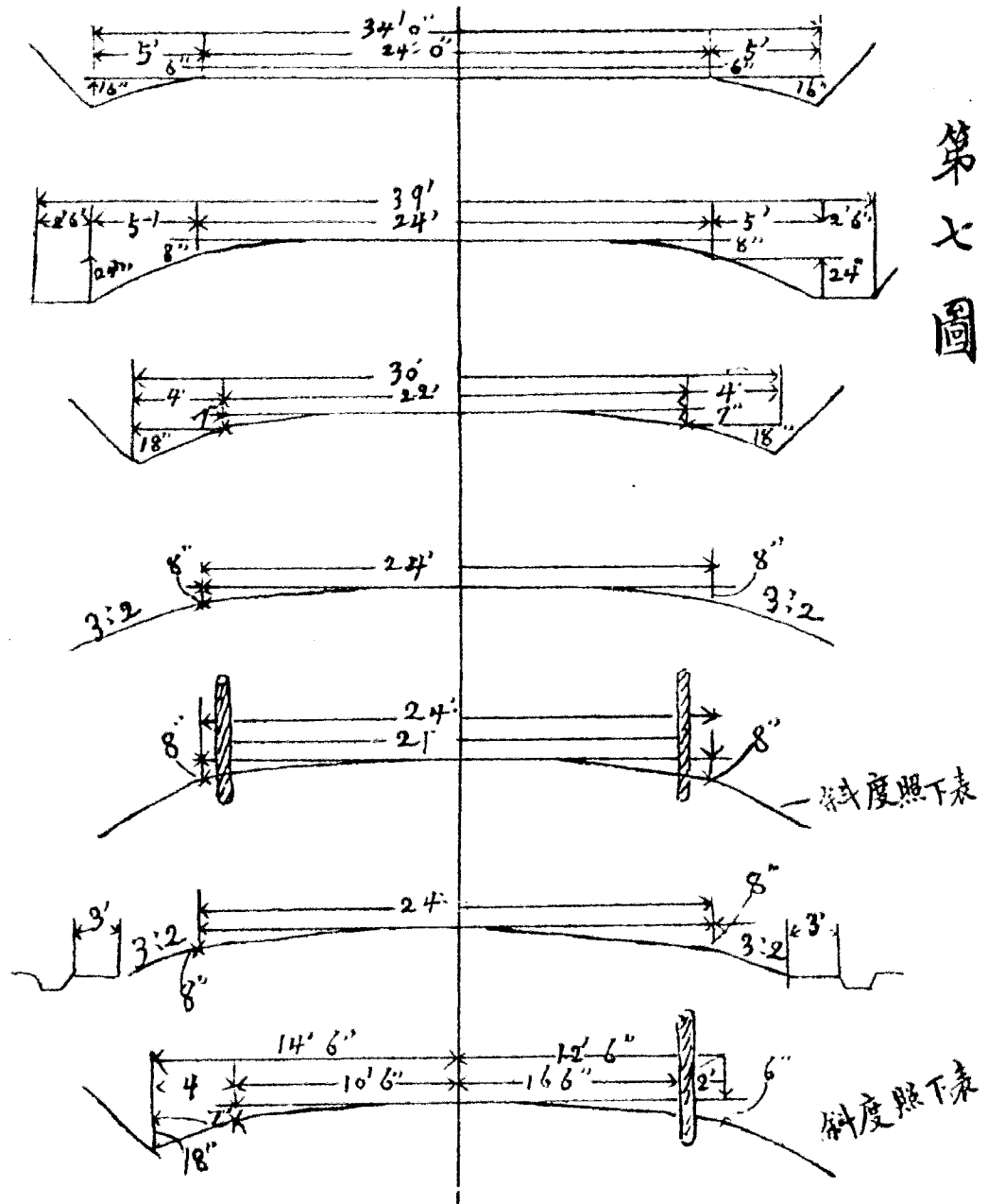
對各種土質所應需之斜度
