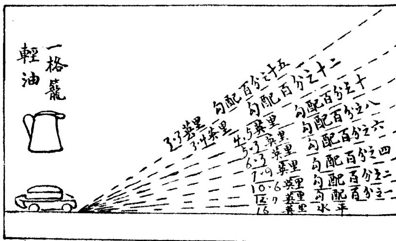
同量一格籠之輕油同勻配之大小其所行里數之影響
