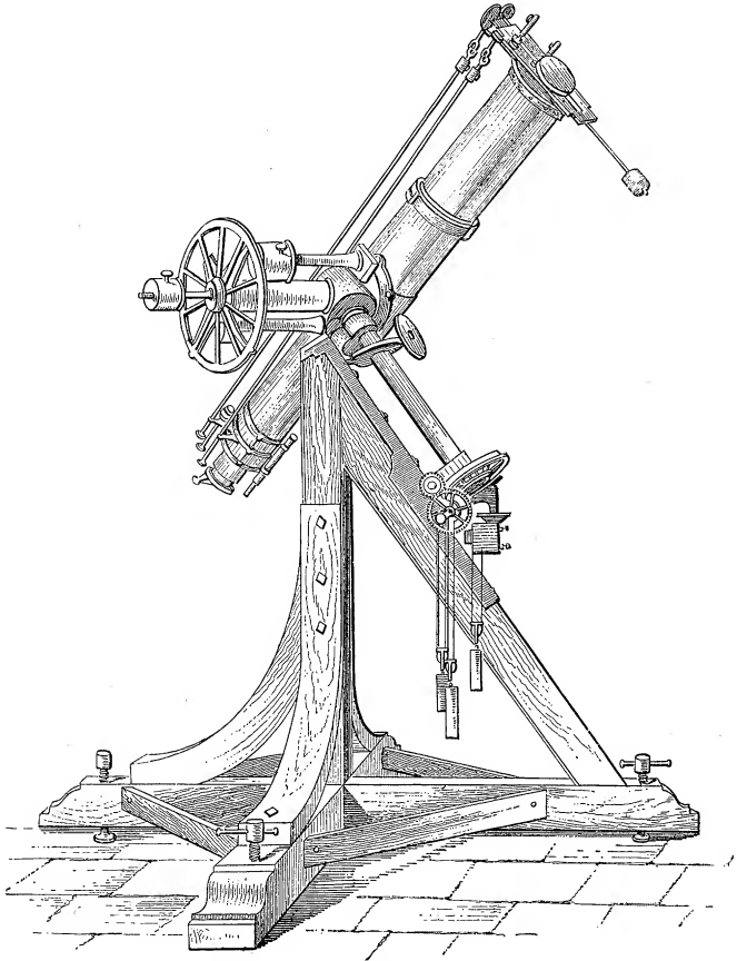
FIG. 92.—Heliometer.
