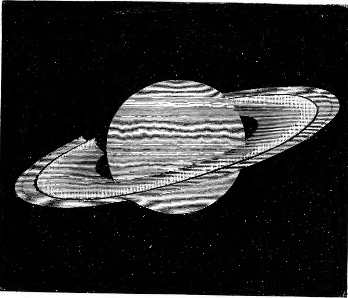
FIG. 81.—Saturn.
