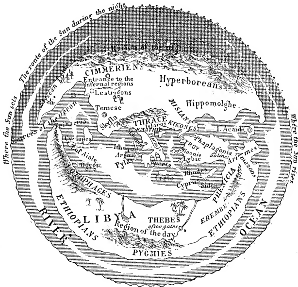
FIG. 4.—Homeric Cosmogony.
