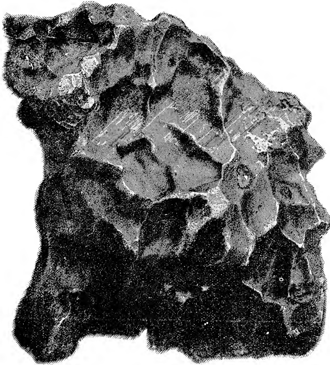
FIG. 95.—Meteorite.
