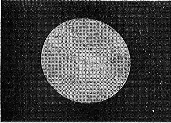
FIG. 72.—Jupiter.
