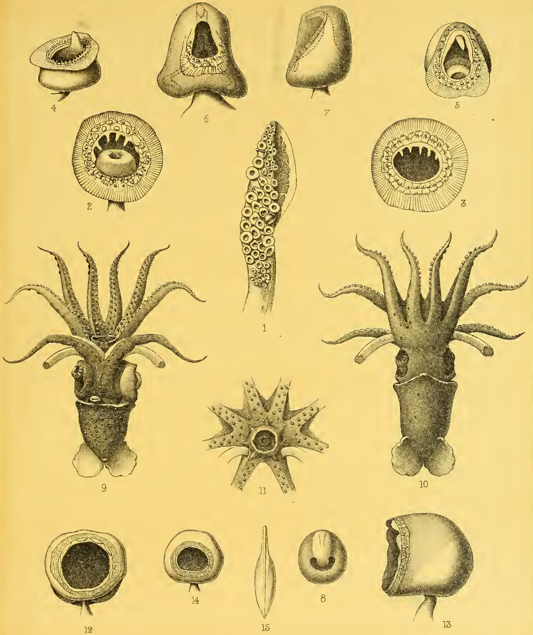
1-8, TELEOTEUTHIS CARIBBÆA (Lesr.) 9-15, HISTIOPSIS ATLANTICA, n. gen., n. sp.
