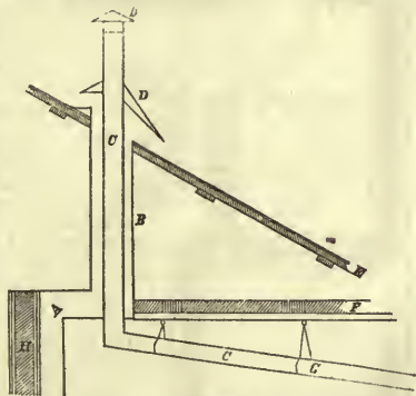
Ventilating Apparatus.
