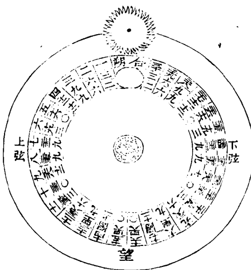
月輪行度圖
