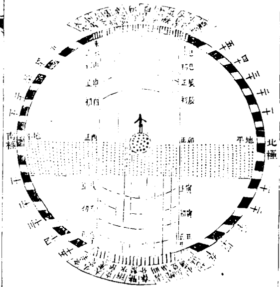
赤道天頂圖
