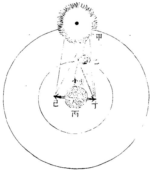
日蝕三差圖
