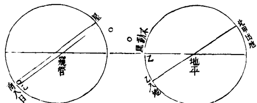
北極圖
