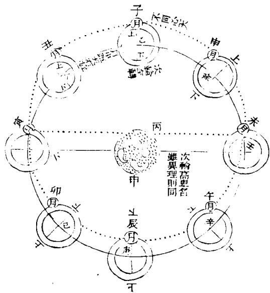
月行次輪圖
