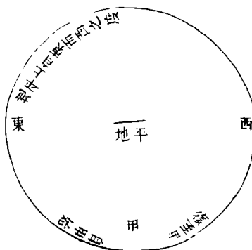
天左旋圖
