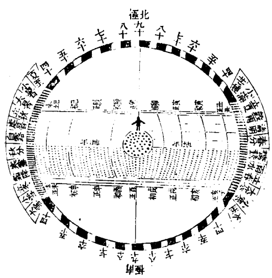
北極天頂圖
