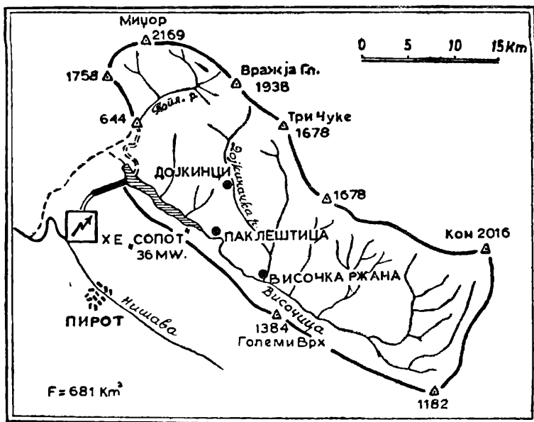
Ск. 2 Карта слива будуће акумулације Завој
