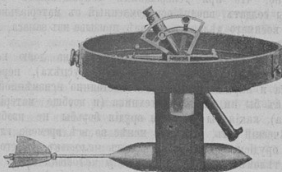
Приборъ Райлей-Скотта для метанія бомбъ. (Къ ст. „Воздушные гренaдеры“).
