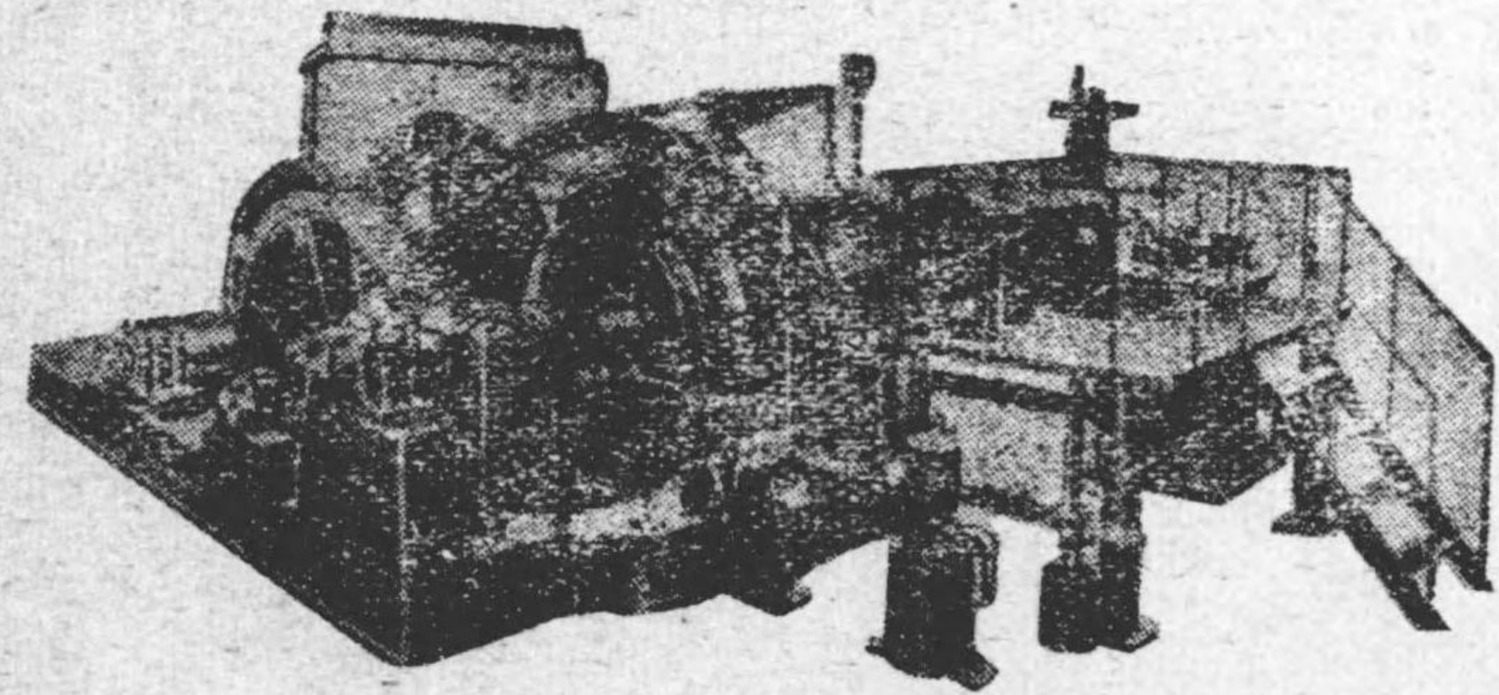
300馬力單胴電氣捲揚機
