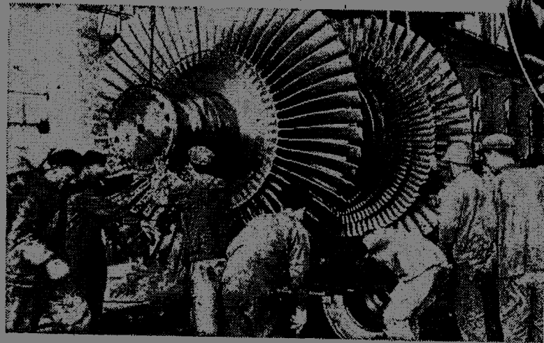
在毛主席“独立自主，自力更生”的方针指引下，我国工人阶级自己设计和制造了赶超世界先进水平的一万五千瓩水冷汽轮机发电机组。因为工人们正在安装汽轮机。 (新华社记者摄)
