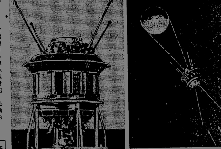
自动月球探测器在月球背面着陆的情况(右下方的箭头表示太阳的方向)。
