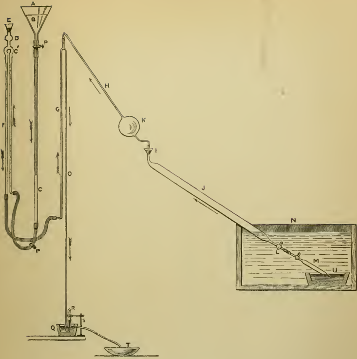
FIG. 199.—Frankland-Sprengel pump (§ 28).
