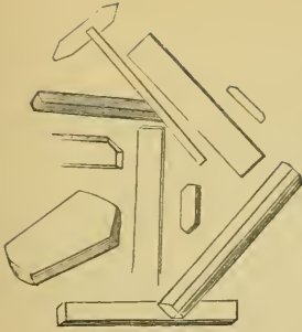
FIG. 322.—Urea.
