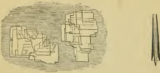
FIG. 314.—Cholesterin.
