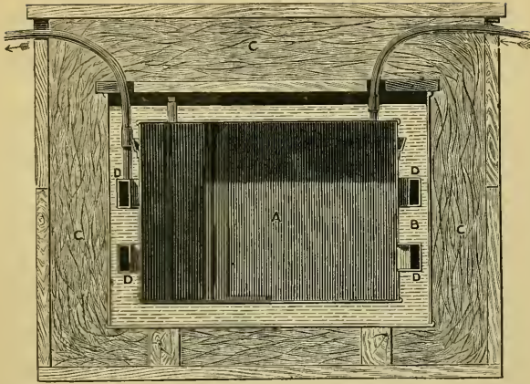
FIG. 265.—The calorimeter (§ 116).
