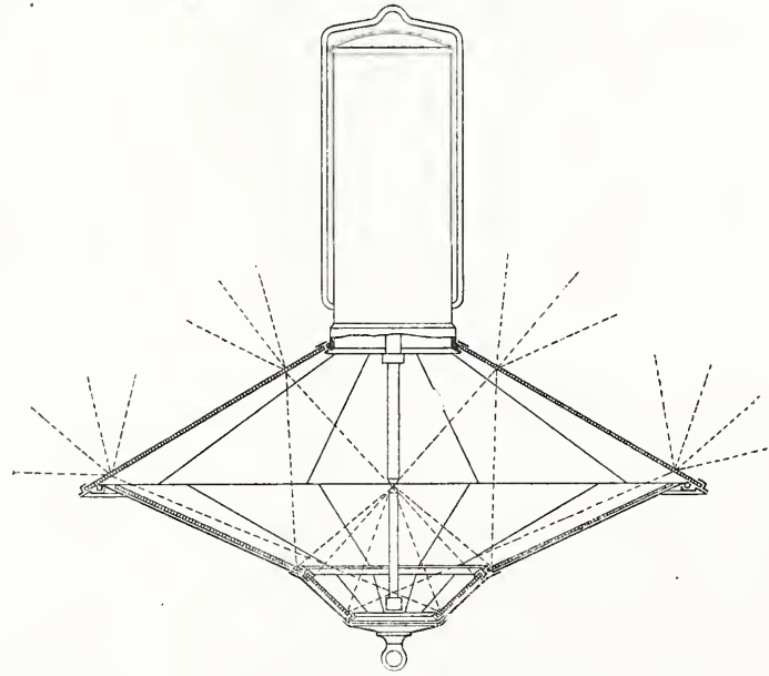
(Fig. 2.) Model voor zalen.
