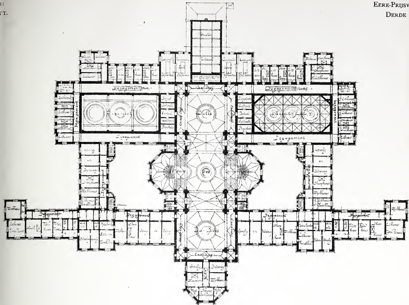
Plan, Eerste Verdieping
