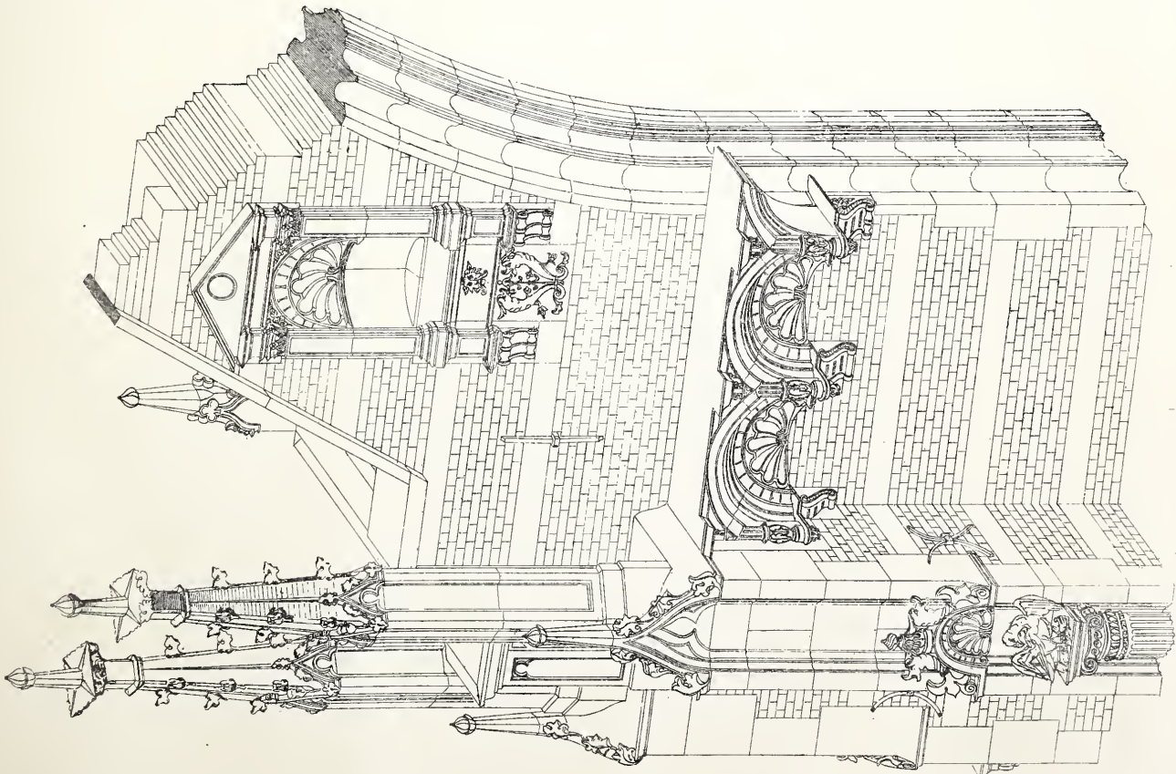
RESTAURATIE NOORDERGEVEL DER NIEUWE KERK TE AMSTERDAM.
