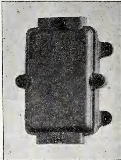
(Fig. 8.) Dubbelpolige loodsluiting voor zeer vochtige ruimten (gesloten).
