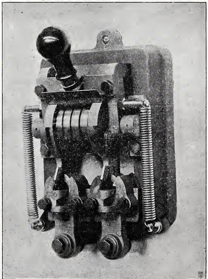
(Fig. 6.) Automatische afsluiter.
