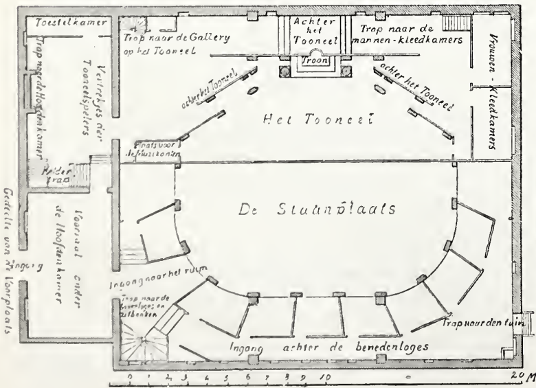
PLATTEGROND van den Schouwburg op de Keizergracht te Amsterdam. Gesticht in 1637.
