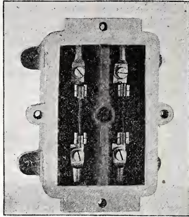
(Fig. 7.) Dubbele loodsluiting voor zeer vochtige ruimten (open).
