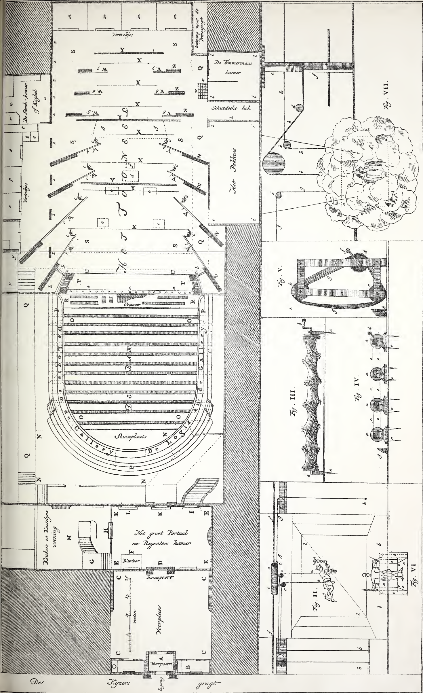
Platte Grond van den gewezenen Schouburg te Amsterdam, zoo als dezelve geweest is voor den Brand van den 11 May 1772, Benevens de Abeelding van eenige Konstwerken.
