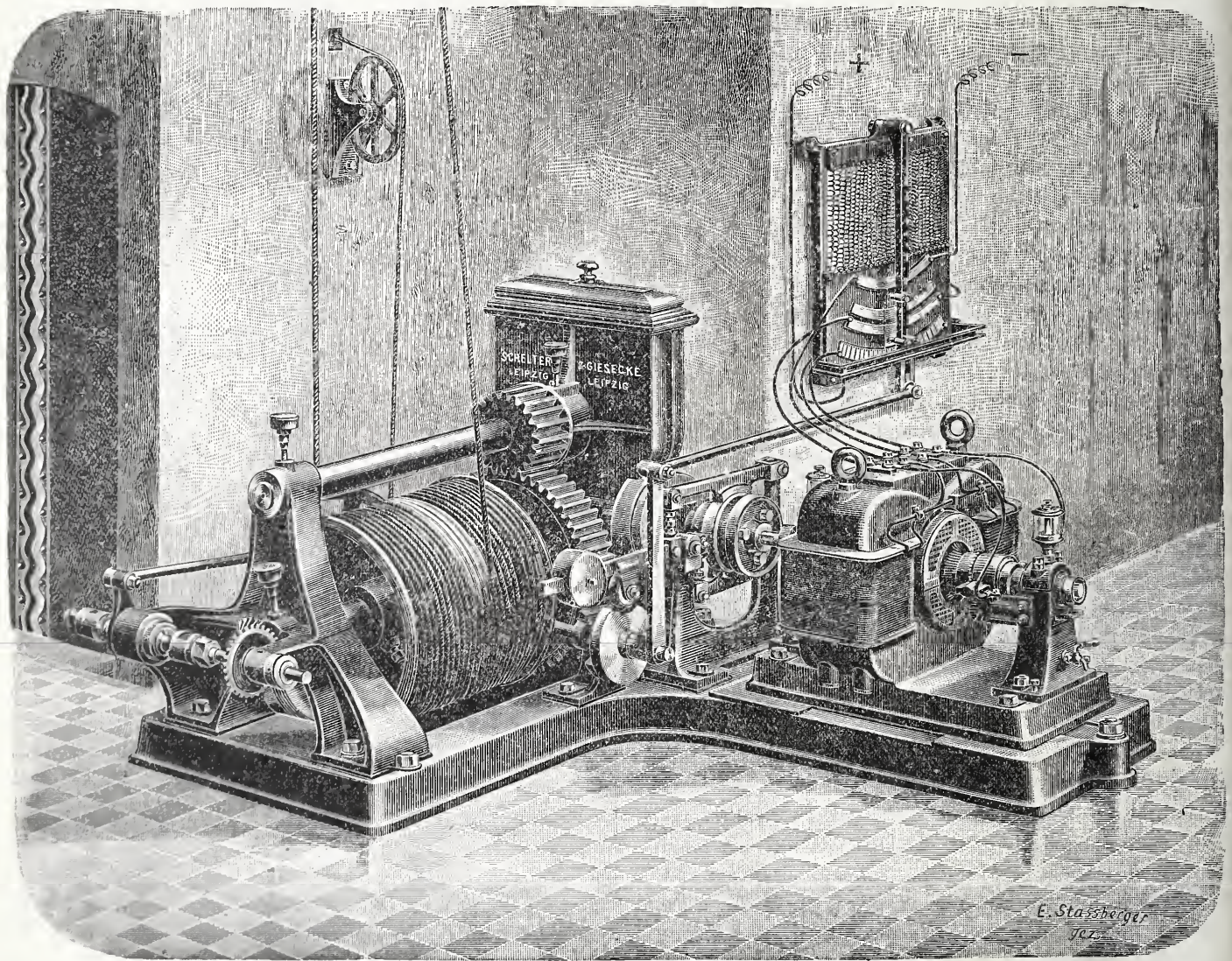
Fig. 1. Hijstoestel.
