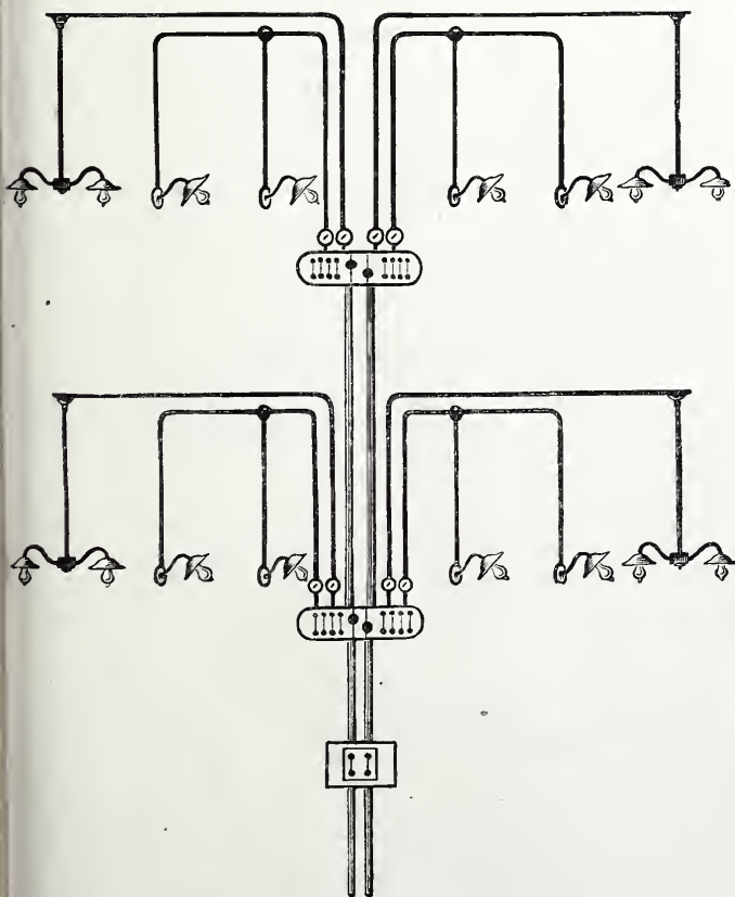
(Fig. 16.) Schema van verbindingen door middel van Bergmannsche buizen.
