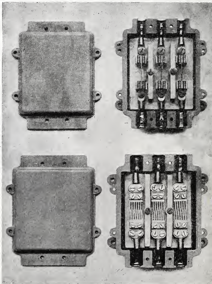
(Fig 9.) Driepolige loodsluitingen voor zeer vochtige ruimten.
