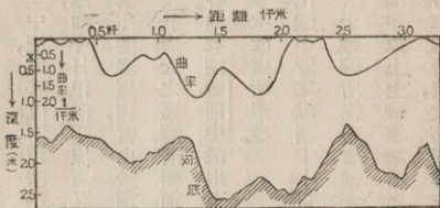
第四一圖 曲率與深水之對照
