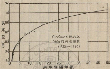
第一三圖 洪水水位與洪水間隔年數(俄亥俄河)
