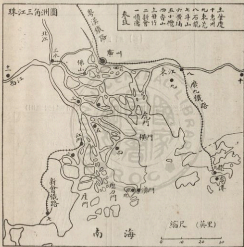
川狀網之洲角三江珠
