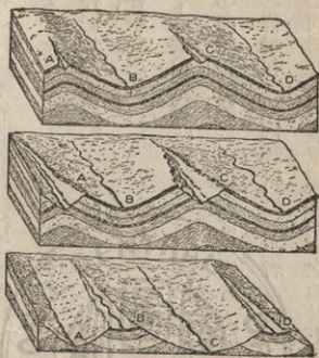
第四八圖 (C.A.)谷斜背與(D.B.)谷斜向 及其發達
