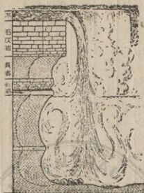
第 二 四 圖 耐 亞 嘎 拉 流 壺 之 渦 捲
