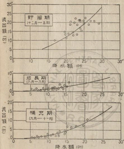
美國降水與水流額之關係 第二圖
