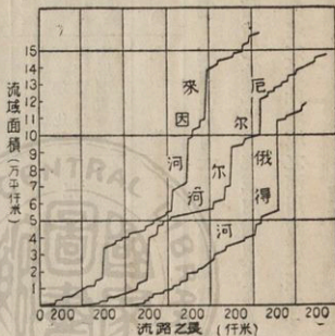
第一圖 流域之平均幅員
