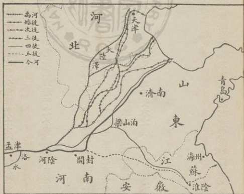
遷變之路流河黃 圖一三第
