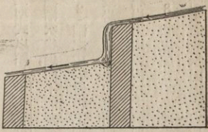
瀧之層岩硬斜傾在懸 圖七二第
