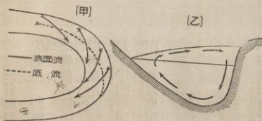
向流之部曲彎 圖九三第
