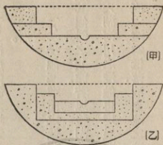
第四四圖 段丘橫斷面之遺
