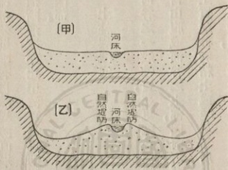
谷河字U種二 圖〇二第
