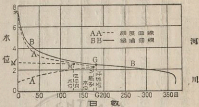
(河伯爾尼)數日與位水 圖五第
