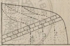
瀧之層岩硬斜傾在懸 圖七二第
