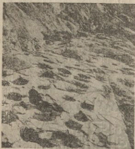
第二二圖 花崗岩之上甌穴
