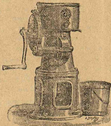
Nona mașina de spălat și scurs untul (a se vedea explicația în acest No.)
