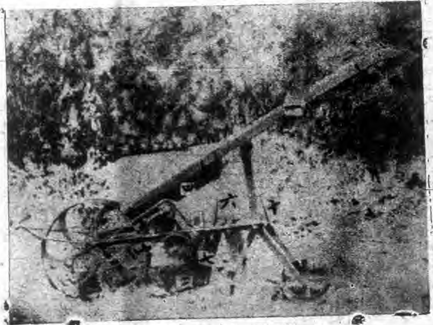
圖 1 一、機柄 二、轆輪 三、開溝器 四、種箱 五、撥種器 六、密度器 七、下種器 八、覆土器 九、壓土器 十、開關器 十一、齒輪 十二、鏈條
