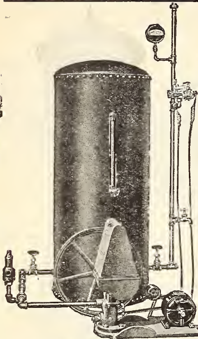
Fig. 1355-A Pump
