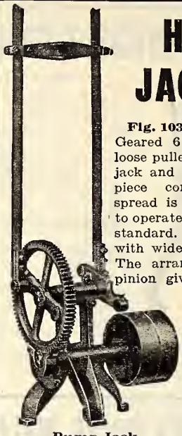
Pump Jack Fig. 1037.
