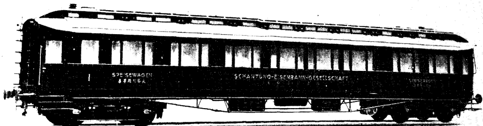
Vierachsiger kombinierter Speise- & Schlafwagen mit Spindel- & Luftdruckbremse, elektr. Beleuchtung, Dampf & Warmwasserheizung, gebaut fuer die Kiao-Tsi-Eisenbahn, China.
