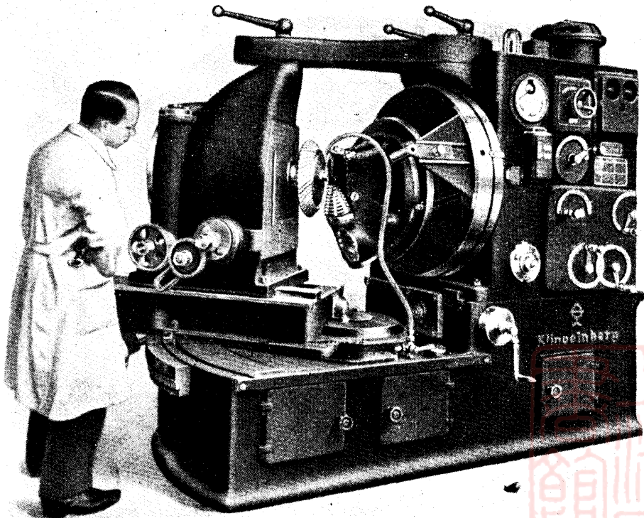
Spiralkegelrad-Abwaelzautomat Mod. FK 200 D.
