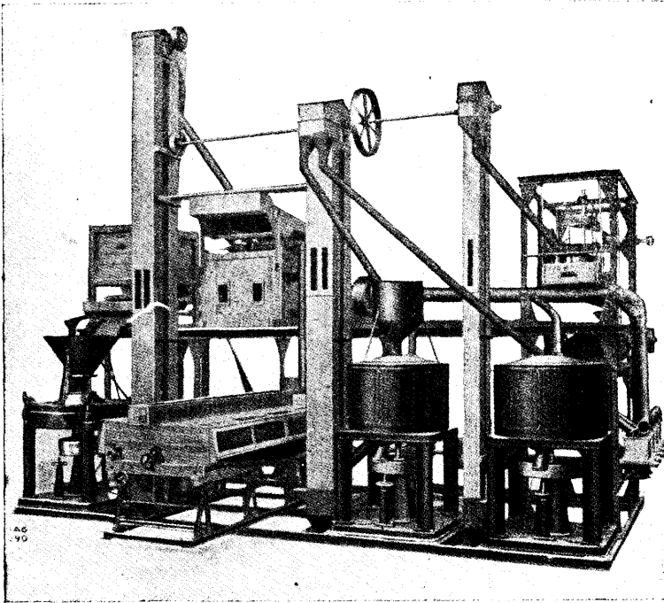
Reismuehle in Kiangsi 廠米碾昌南
