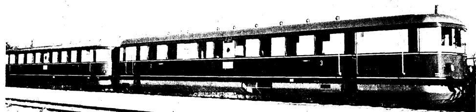
410 PS diesel-elektrischer Triebwagen, 100 km/Std. Geschwindigkeit, mit Maybach-Motor & elektr. Kraft-uebertragung B.B.C.
