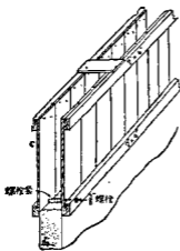
第十四圖 牆之活動板型
