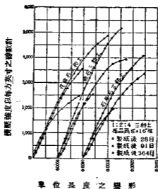
第二十二圖 三和土受擠壓時之應力變形圖
