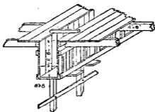
第十三圖 梁之板型
