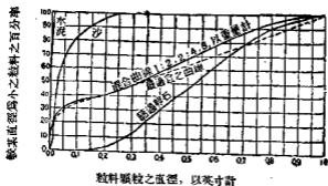
第五圖 粗細粒料之細度分析曲線
