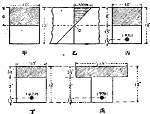
第二十五圖 三和土梁之設計
