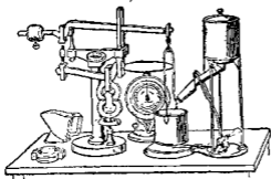
第四圖 水泥膠沙牽引強度試驗機
