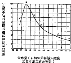
第十九圖 三和土擠壓強度與含水量之關係
