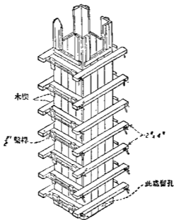
第十二圖 柱之板型用直板作成
