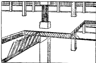
第二十七圖 卡氏式之梁及柱中鋼骨布置之情形
