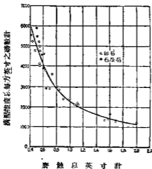
第二十三圖 三和土腐蝕深度與抵抗腐蝕性之關係
