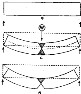
第二十四圖 梁之受力情形
