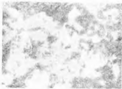
第一圖 砂岩
