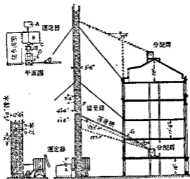
第十圖 美國國立印刷局建築工場三和土布置情形
