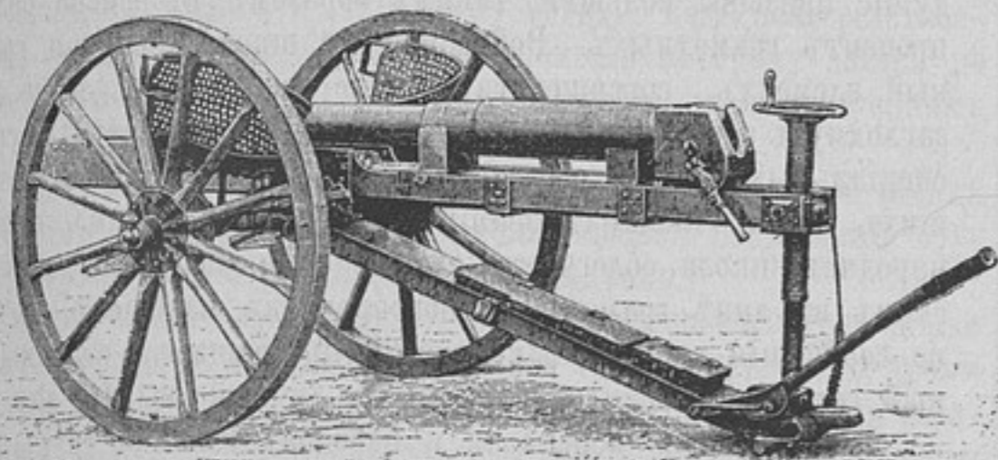
№ 4. Полевое скорострѣльное орудіе послѣ выстрѣла; тѣло орудія искусственно удержано въ крайнемъ положеніи отката.
