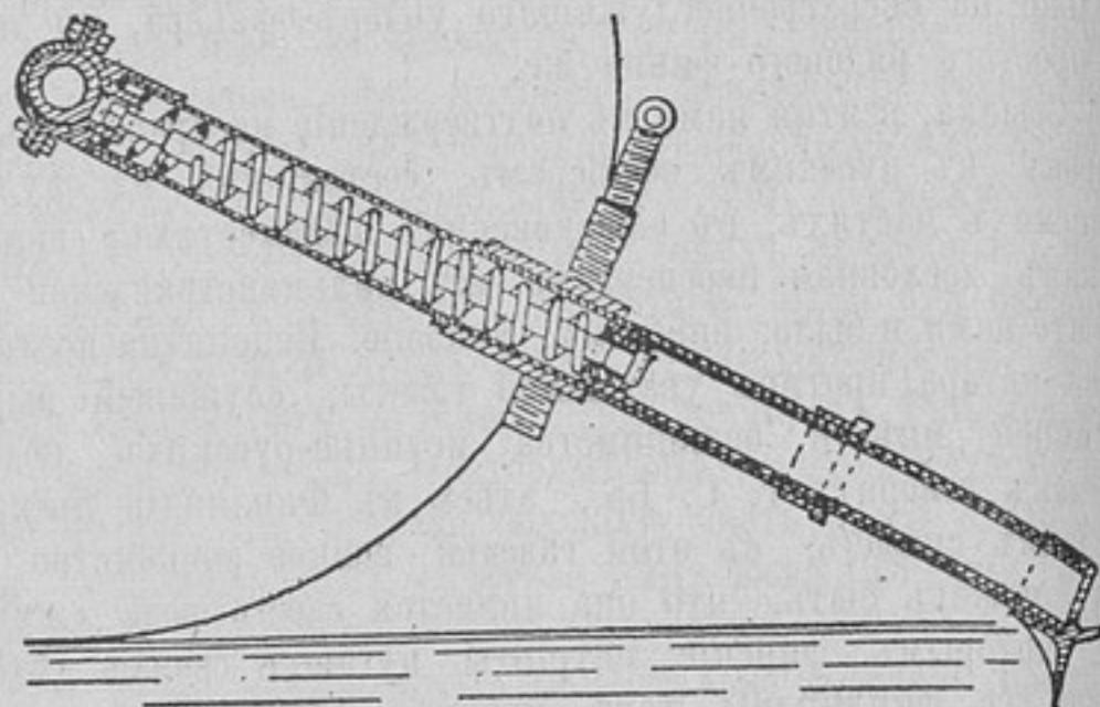
№ 1. Схематическій чертежъ телескоп-лафета.
