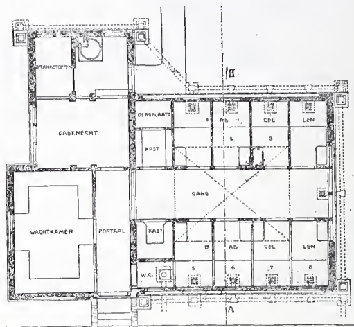
Plattegrond. Schaal 1 à 200. Badhuis voor Volksbaden. Ontwerpers: J. H. W. LELIMAN EN FIRMA ROBERT KALFF EN CO.
