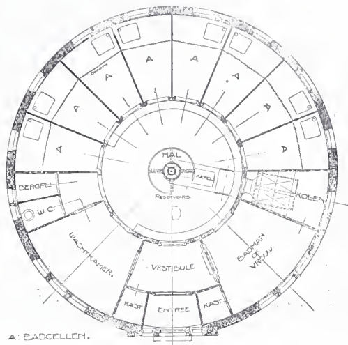
Plattegrond. Schaal 1 à 200. Badhuis voor Volksbaden. Ontwerper: JOH. VAN ASPEREN.
