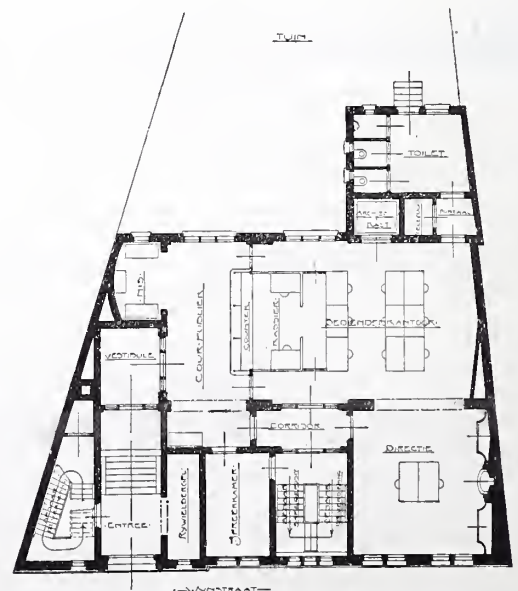
Plattegrond. — Schaal 1 op 300.
