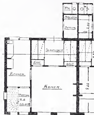
Plattegrond.
