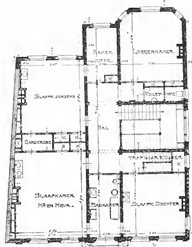
Eerste verdieping. schaal 1 à 300.
