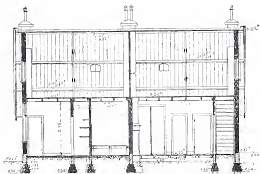
Doorsnede C-D.
