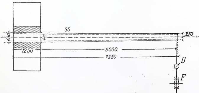
Fig. 8. Bevestigde mast voor de proefneming.
