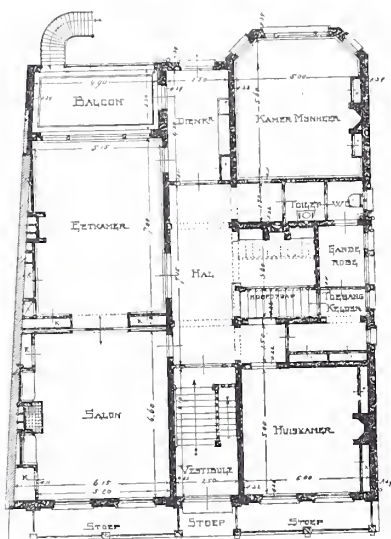
Bel-étage.
