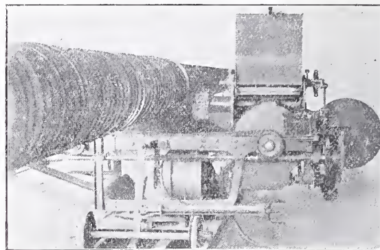
Fig. 3. Bewapenen der masten.
