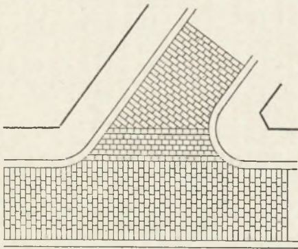
Рис. 3. Расположеніе брусковъ на углу 2-хъ улицъ.
