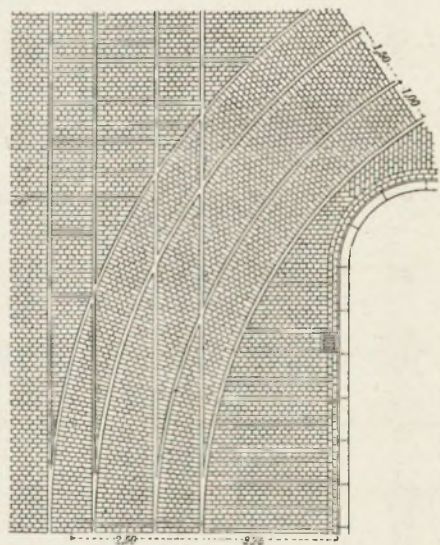
Рис. 2. Укладка брусковъ между путями.
