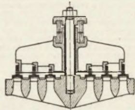
Фиг. 8. Многослойной клапанъ.
