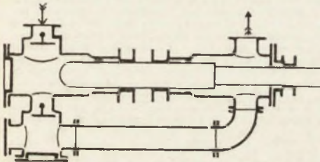
Фиг. 7. Схема дифференціального дѣйствія.
