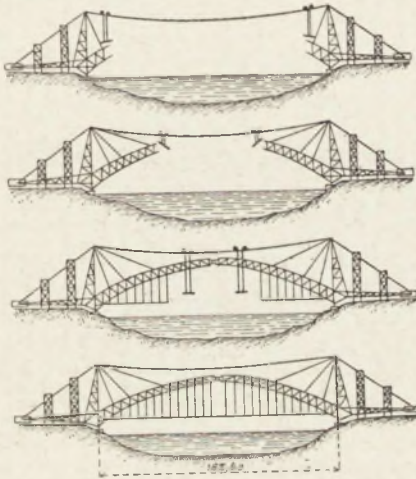
Рис. 19. Сборка на вѣсу.
