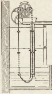
Фиг. 3. Цѣнное колесо.
