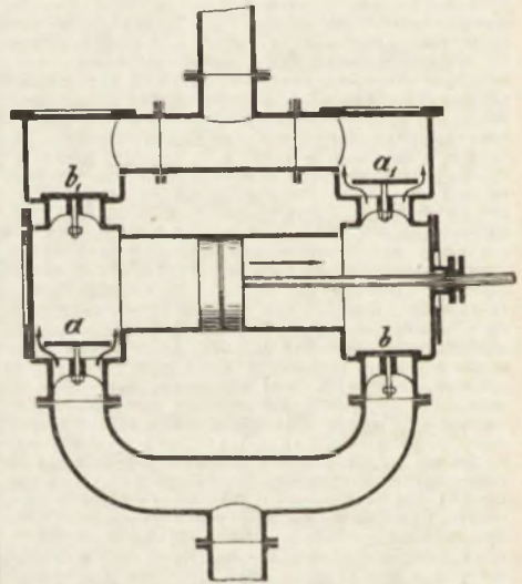
Фиг. 5. Схема насоса двойного дѣйствія.
