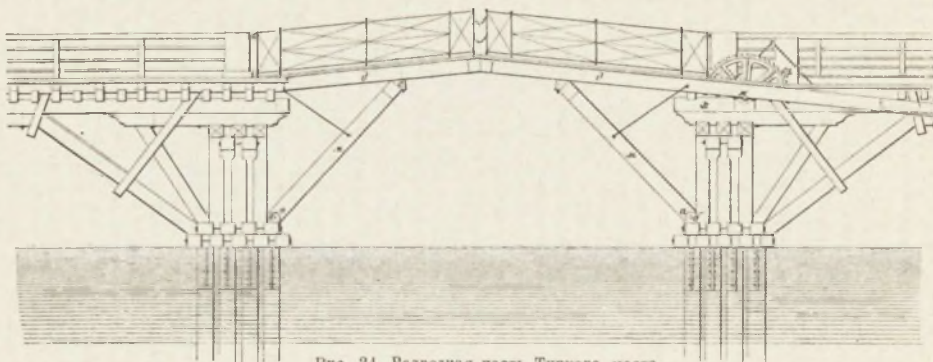
Рис. 24. Разводная часть Тучкова моста.
