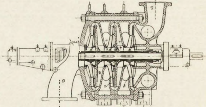
Фиг. 16. Центробежный насосъ многоступенчатый.
