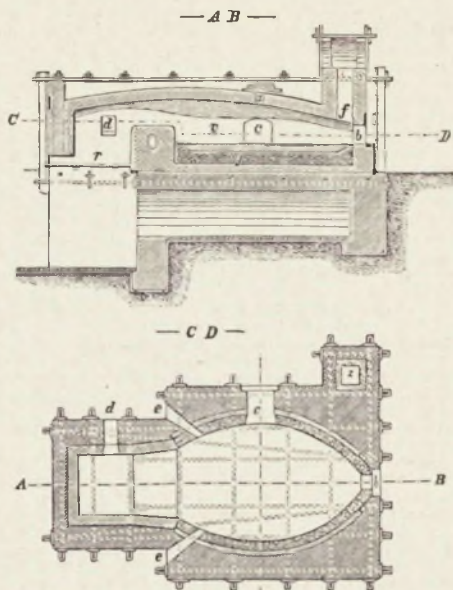
Рис. 9. Пламенная печь для рафинированія черной мѣди. Первый видъ — продольный вертикальный разрѣзъ печи; второй — продольный горизонтальный по уровню пода печи. в — нагрѣвательная камера съ подомъ, сдѣланнымъ изъ кварца; г — колосниковая рѣшетка для сжиганія угля; д — шуровальное отверстіе; ф — дымовой каналъ; е — каналы для впуска окислительнаго воздуха въ нагрѣвательную камеру; а — отверстіе въ сводѣ для впаденія мелочи; с — садочная печь для большихъ кусковъ; б — рабочее отверстіе; з — дымоходъ. Рафинированная мѣдь вычерпывается черезъ рабочее отверстіе б .
