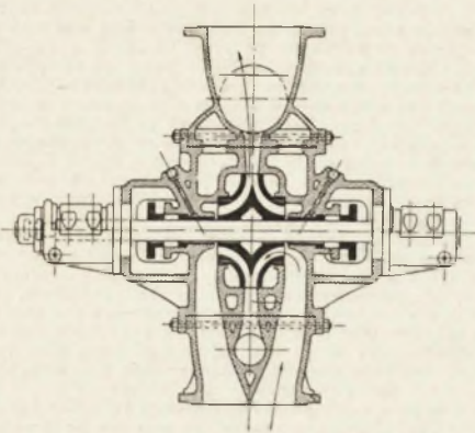
Фиг. 15. Центробежный насос двоярный.
