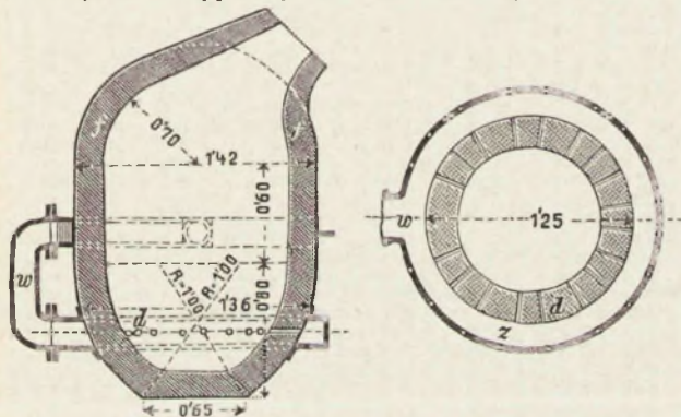
Рис. 8. Бессемеровская реторта для выплавки черной мѣди. Направо — вертикальный разрѣзъ; направо — горизонтальный разрѣзъ по сопламъ д , черезъ которыя подается воздухъ въ реторту черезъ расплавленный купферштейнъ. в — коробка для подаваемого воздуха. Реторта изготовляется изъ желѣзныхъ клепаныхъ листовъ; внутри имѣетъ огнеупорную (кварцевую) футеровку г .
