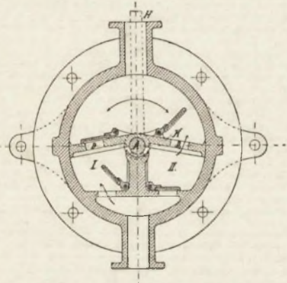
Фиг. 11. Насосъ съ крыльчатымъ поршнемъ.
