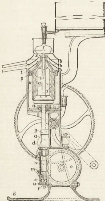
Рис. 4. f —поплавокъ, x —сливочный вѣнтъ, y —проходъ снятого молока, t —резиное кольцо, p —мѣсто свинчиванія двухъ частей барабана, q —центральная крышка, g , h —части горловой муфты, u —обхватъ веретена, a —веретено, d —штифтъ оси, l —гайка, c —булка оси, n —червячная передача, m —смазывательное отверстие, e —головка подшипника, u —шайба подшипника, r —гайка подшипника, o —зубчатое колесо, ö —подставка.
