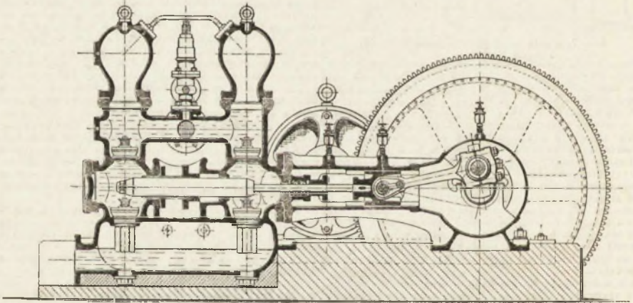
Фиг. 9. Насосъ быстроходный.
