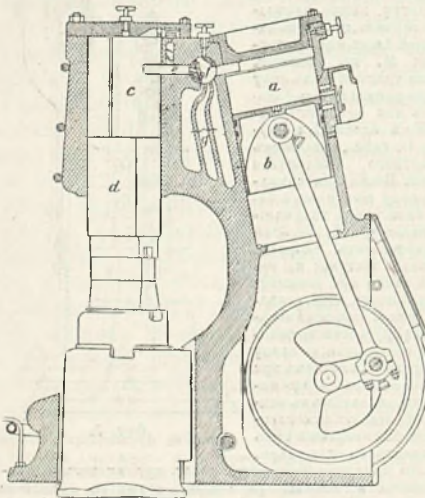
Фиг. 4. Молотъ Іеаклей.
