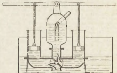
Фиг. 6. Пожарная труба
