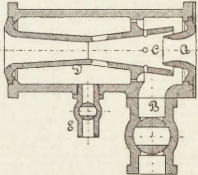
Фиг. 17. Инжекторъ.
