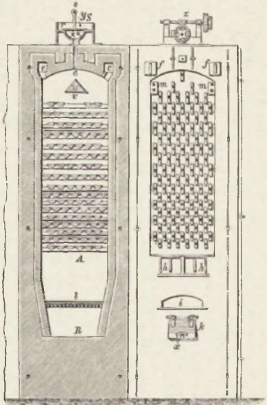
Рис. 4. Печь Герстенберга для порошковой руды. Она состоитъ изъ шахты А, снабженной треугольными балками изъ огнеупорной глины. Шахта предварительно накаливается отъ сжиганія твердаго топлива (угля, дрова). Порошкообразная руда подается изъ ящика З по канаву а при помощи питательныхъ вальцевъ и падаетъ въ шахту на распределительную балку е, сползаетъ по обѣ стороны на слѣдующій рядъ балокъ и т. д.
