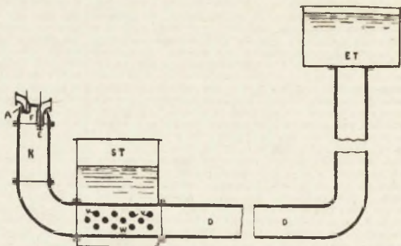
Фиг. 10. Схема насоса Хемфри.
