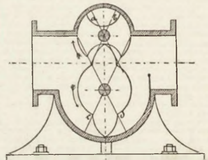
Фиг. 12. Колодратный насосъ.
