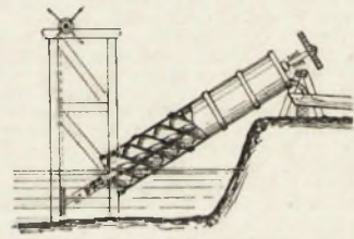
Фиг. 2. Архимедов винт.
