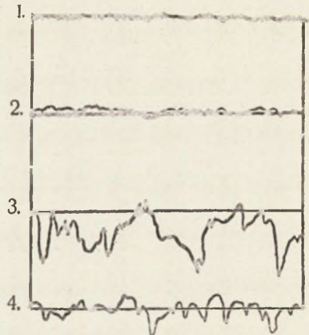
Рис. 1. Кривая 1 относится къ асфальтовой мостовой 2—къ деревянной торцовой, 3—къ каменной брусчатой, 4—къ щебеночной одеждѣ.
