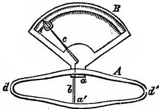
FIG. 24. DYNAMOMETER.
