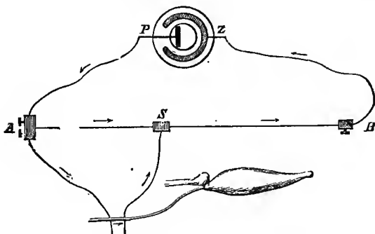
FIG. 32. RHEOCHORD.
