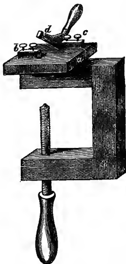
FIG. 14. TETANISING KEY OF DU BOIS-REYMOND.
